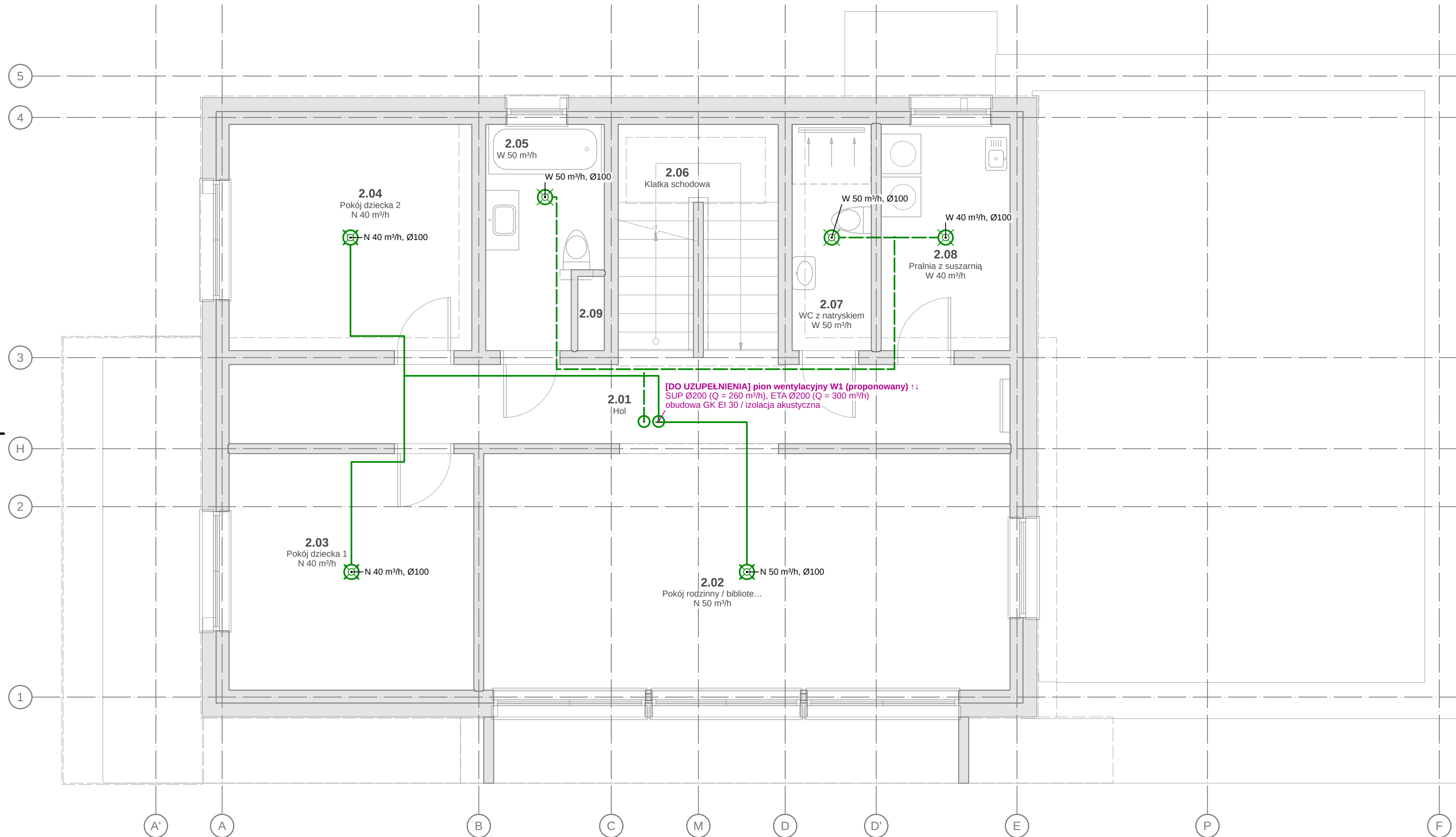
WENTYLACJA MECHANICZNA — RZUT I PIĘTRA 1:50
