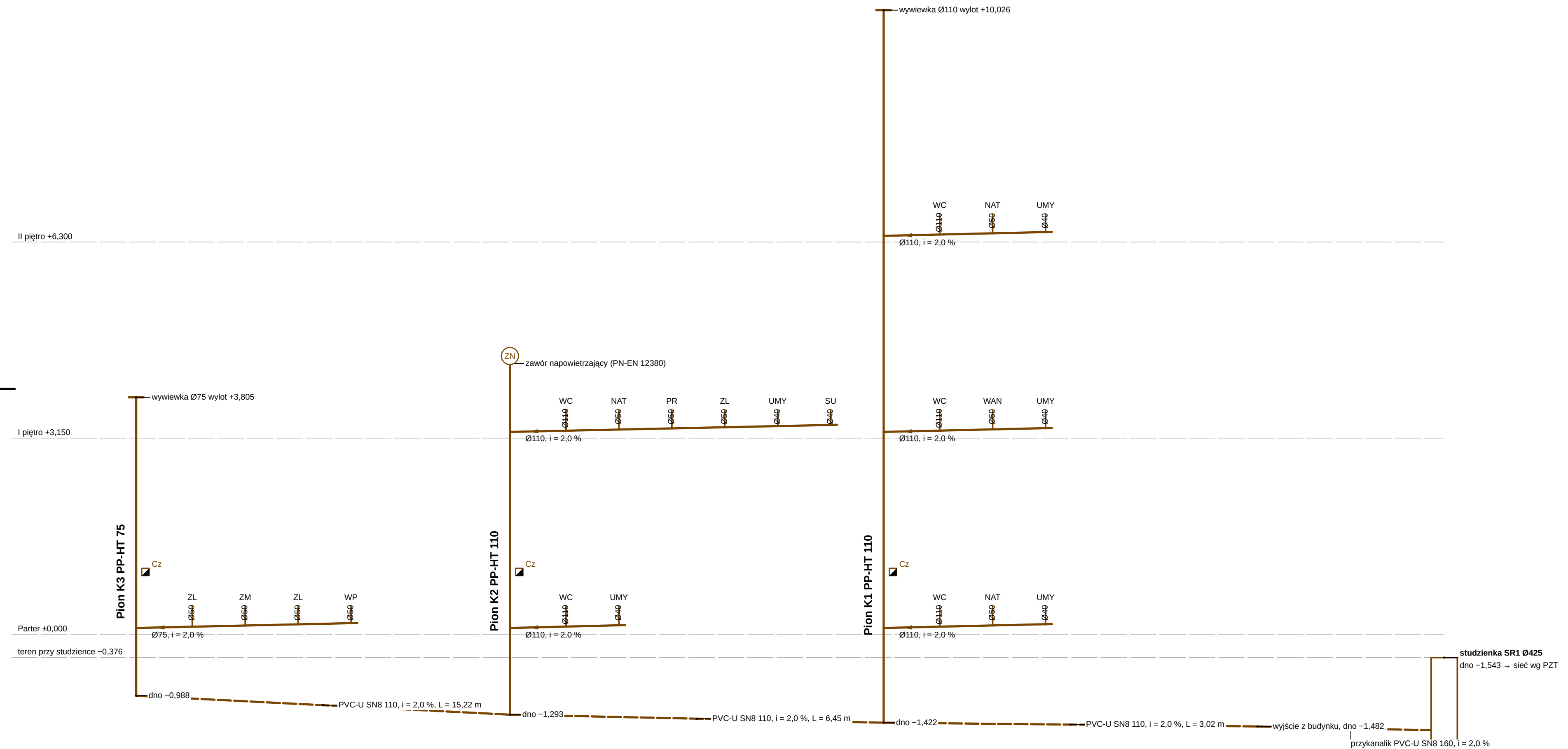
ROZWINIĘCIE KANALIZACJI SANITARNEJ (PIONY)
