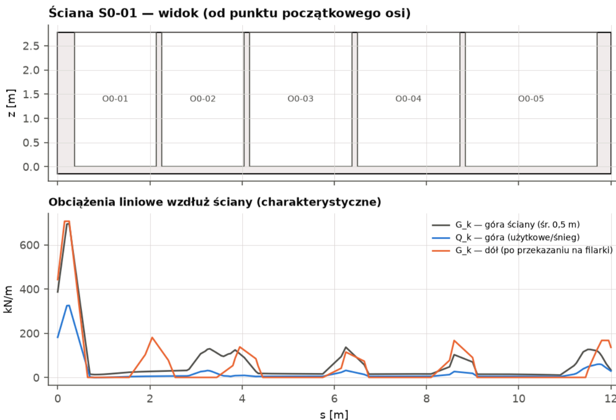
Ilustracja 73. Ściana S0-01: widok z otworami i rozkład obciążeń charakterystycznych wzdłuż osi.
