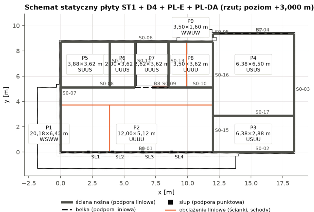
Ilustracja 26. Schemat statyczny płyty ST1 + D4 + PL-E + PL-DA: pola (P — wymiary, warunki brzegowe x=0/x=l , y=0/y=l ; S — podparcie swobodne, U — ciągłość/utwardzenie, W — brzeg swobodny/niepełny), podpory.
