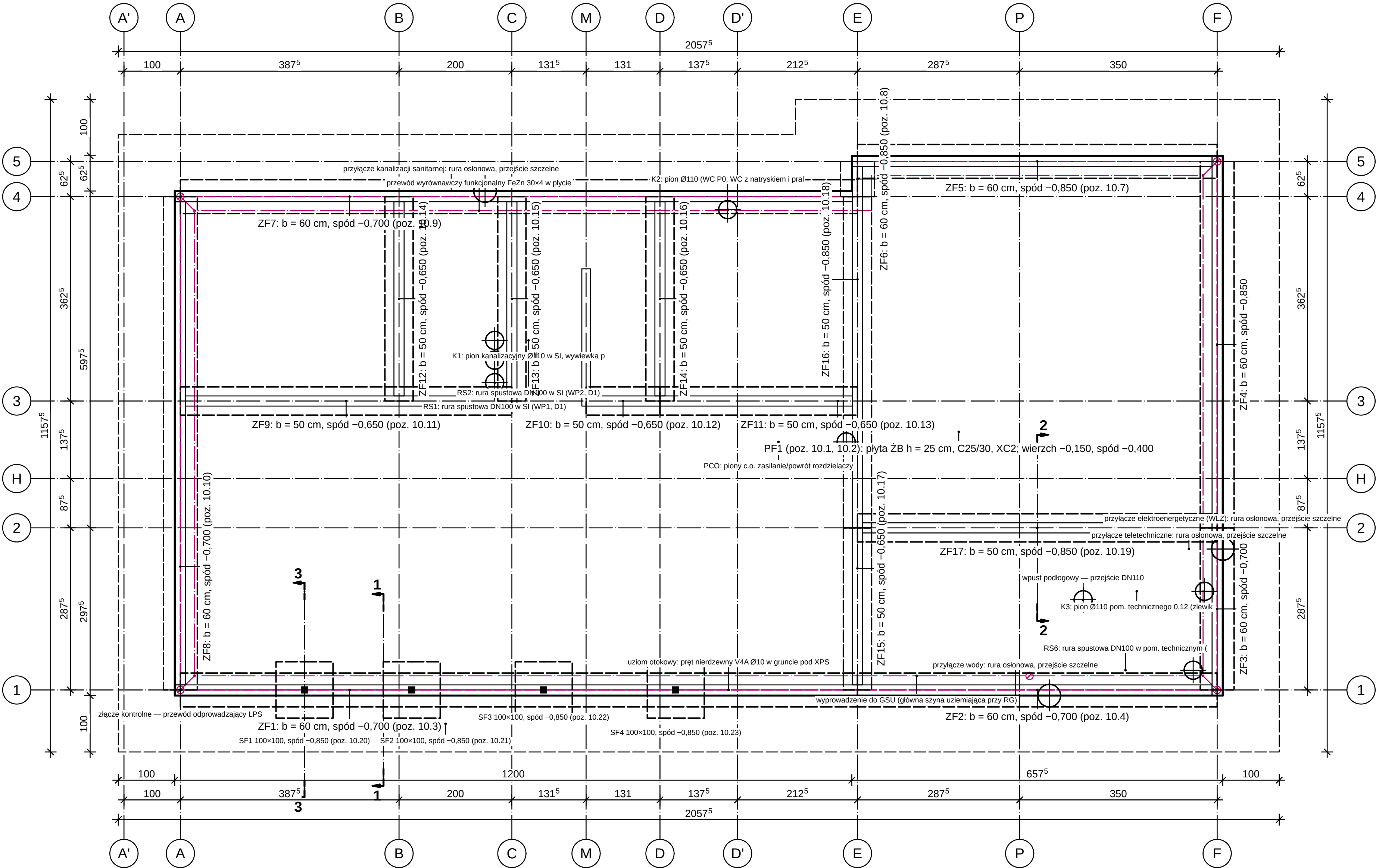
RZUT FUNDAMENTÓW 1:50
