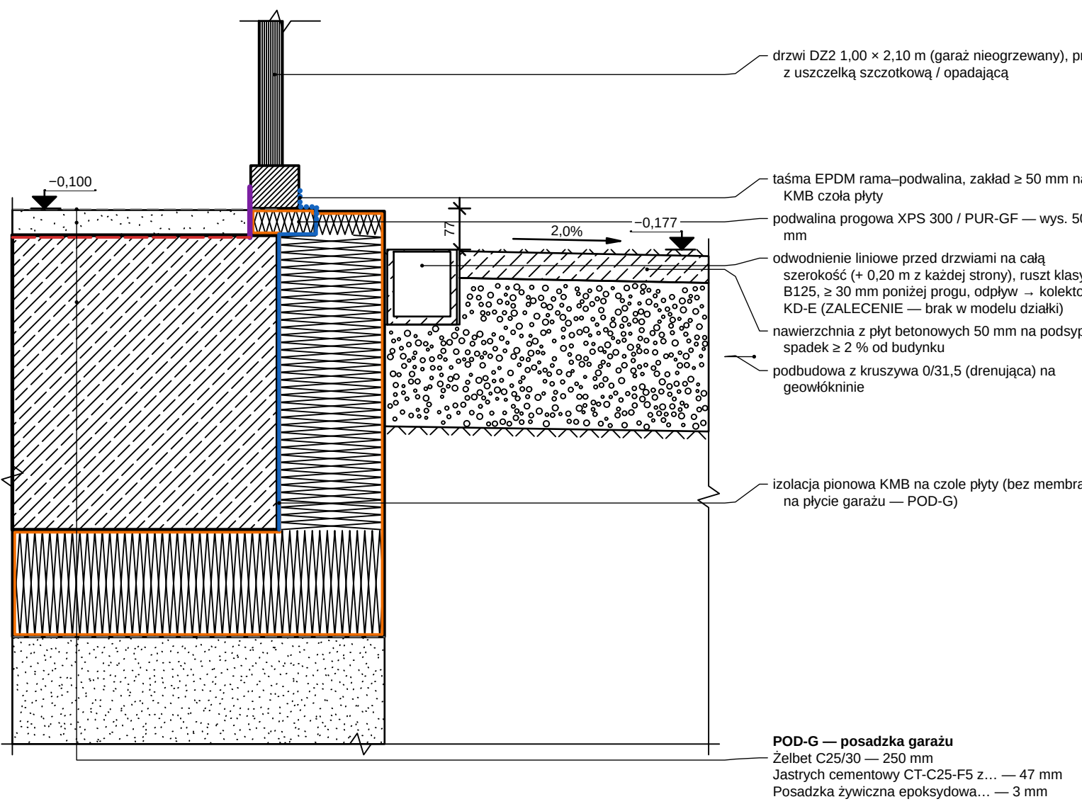
Wzetał bez karty mostka 2D (mostek punktowy / element systemowy) — patrz uwagi 4 linie: H OK, S OK, P OK, I OK — ciągłość zachowana
