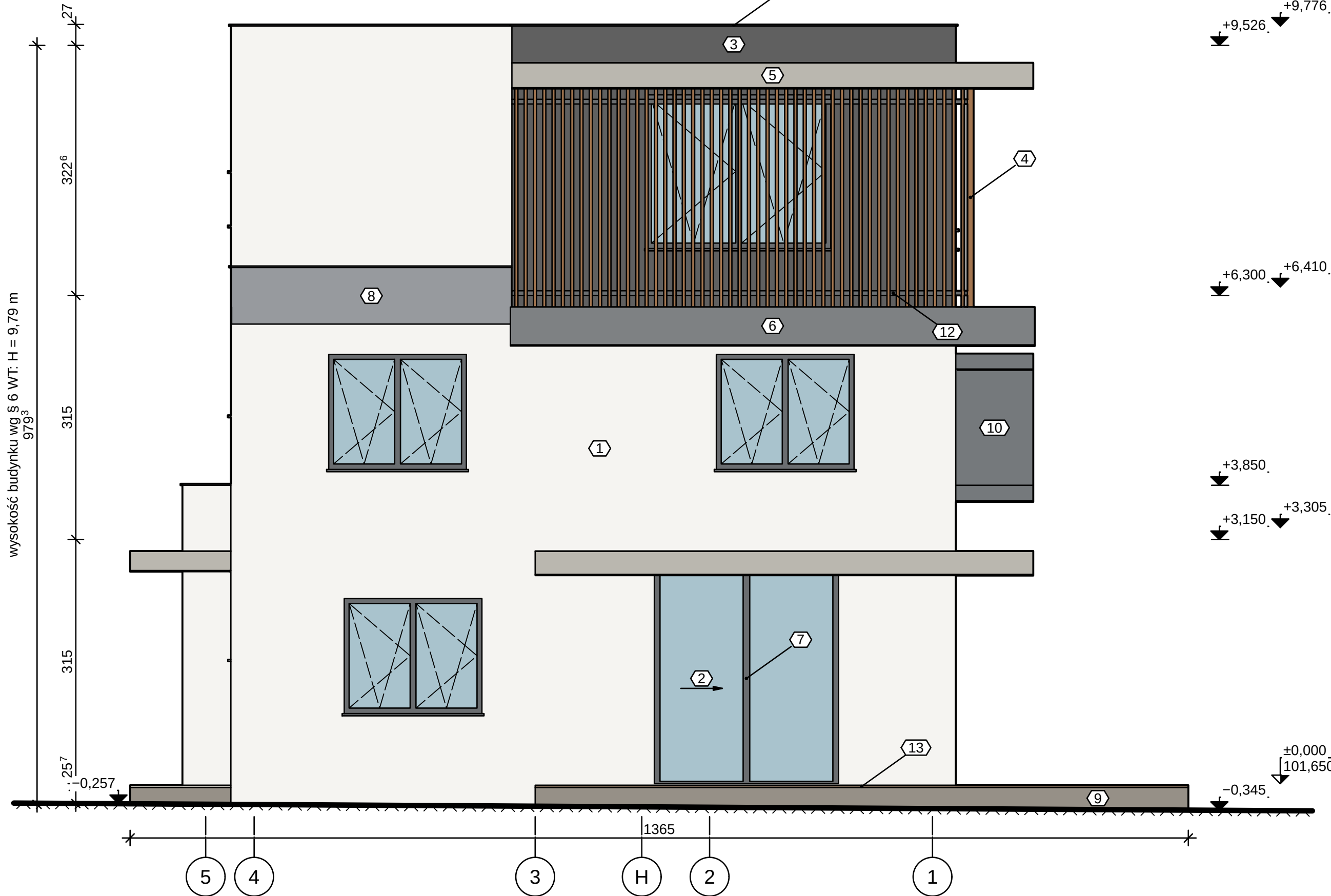
ELEWACJA ZACHODNIA 1:50
