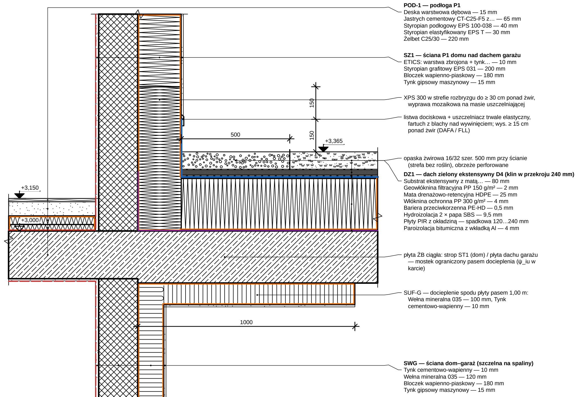
WZ-09c: \psi_e = 0,070 , \psi_{oi} = 0,081 W/(m·K); f_{Rsi} = 0,885 \pm 0,72 — ZLY 4 linie: H OK, S OK, P OK, I uwagi I: WZ-09c: przetrwana: TYNK_GIPS — SIL18 — ZB_C25 (płyta ciągła do strefy nieogrzewanej) — mostek konstrukcyjny; obrys izolacji: 3 części (w tym warstwy dodatkowe...)
