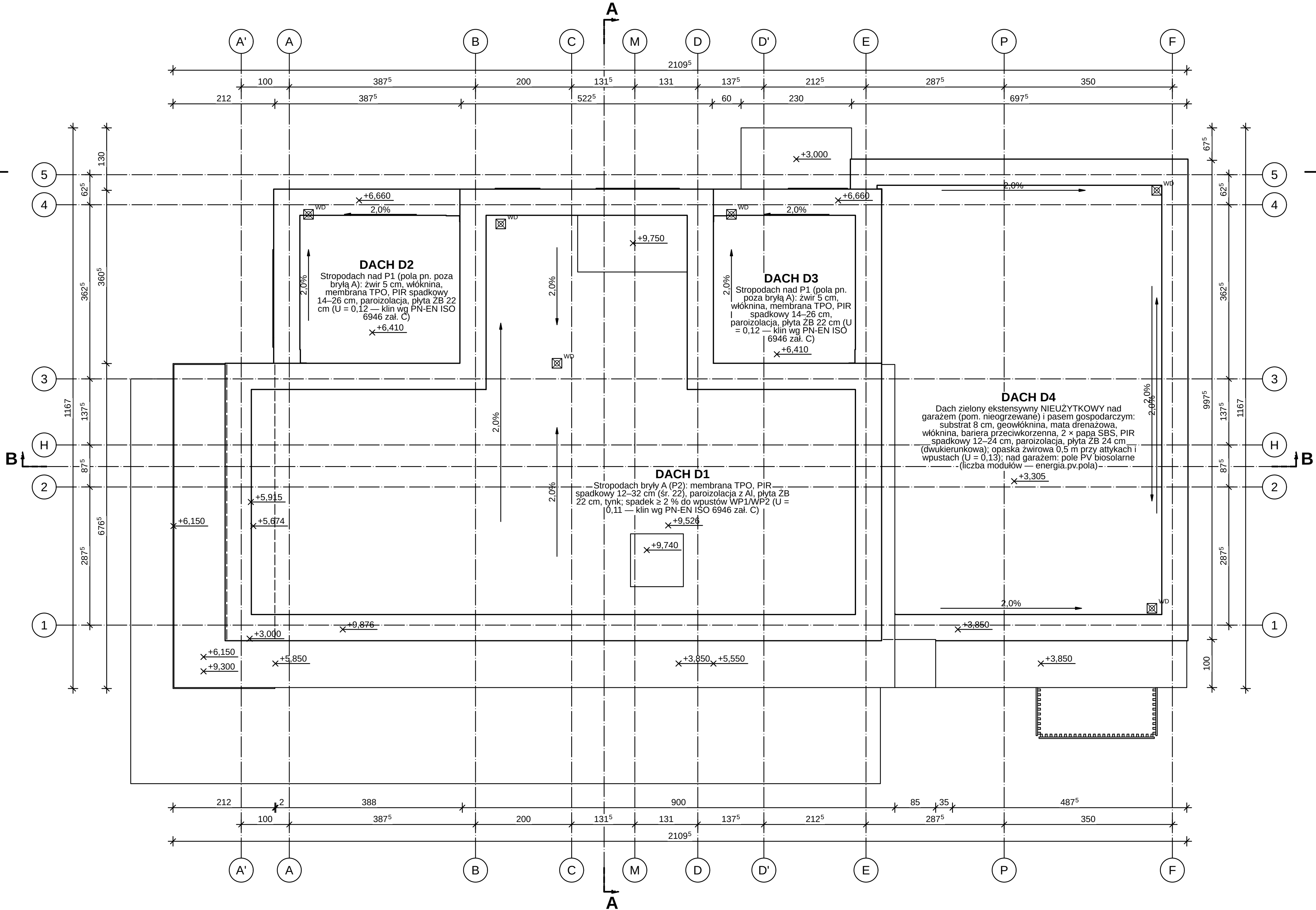
RZUT DACHU 1:50
