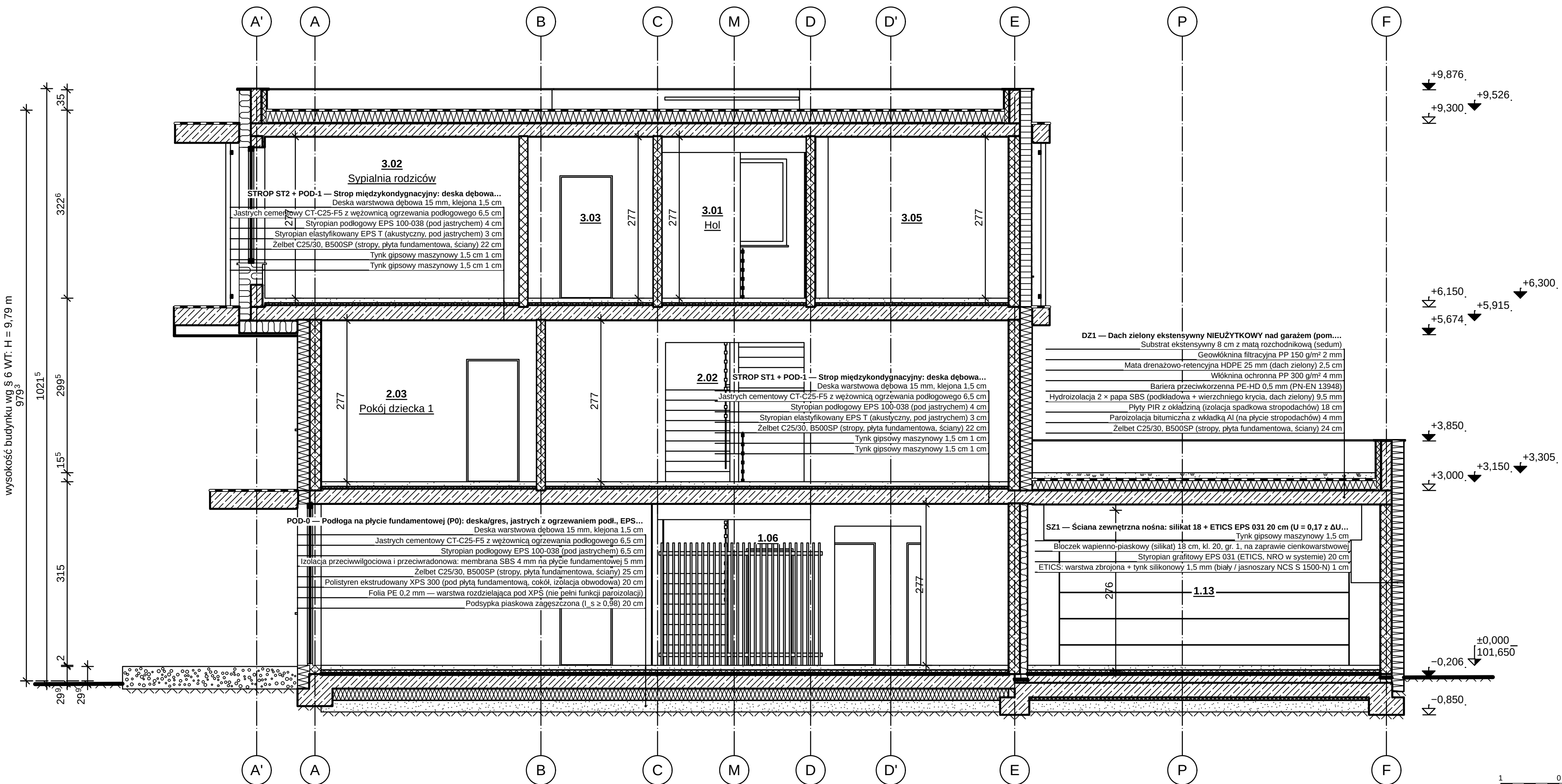
PRZĘKRÓJ B-B 1:50
