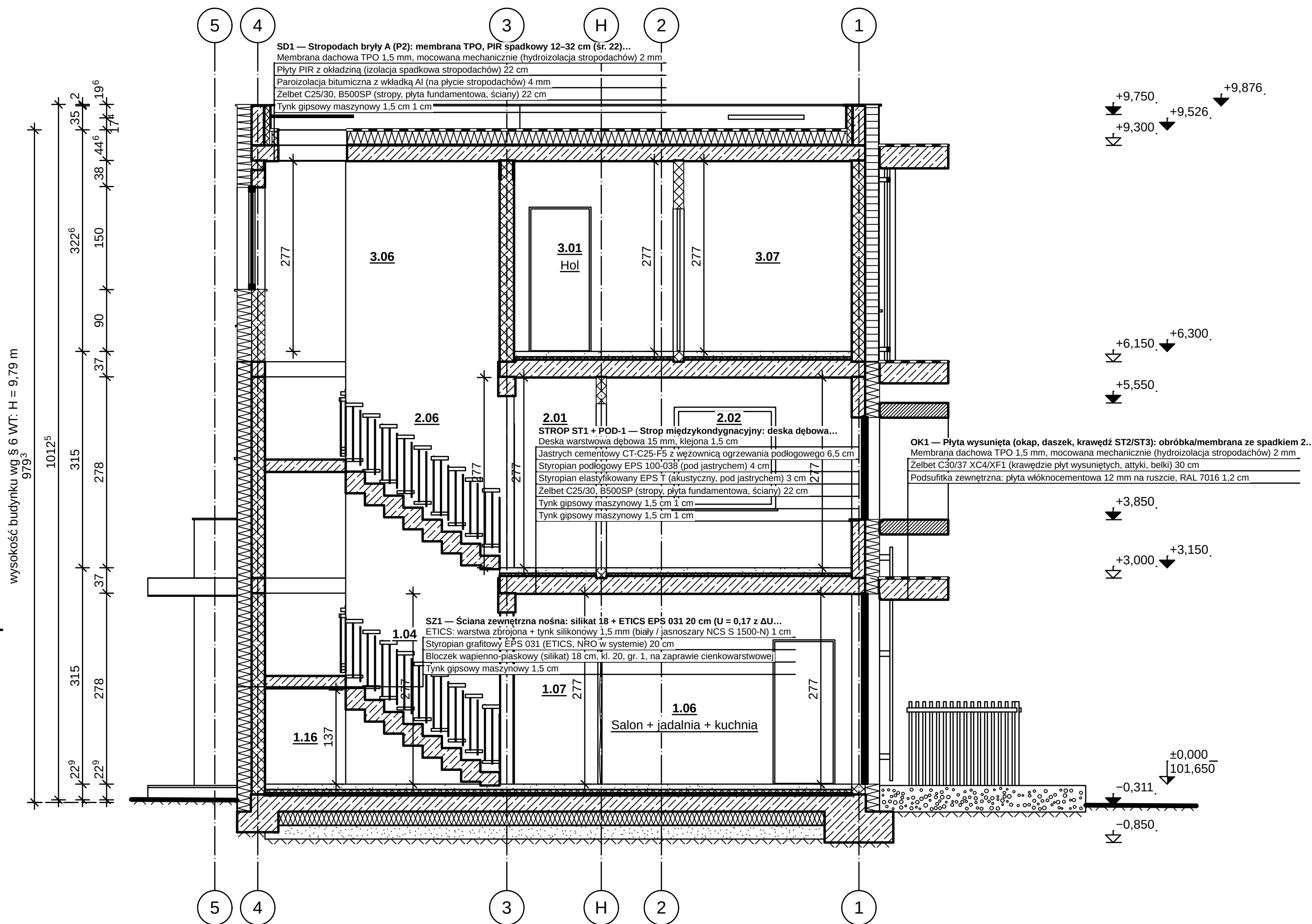
PRZĘKRÓJ A-A 1:50
