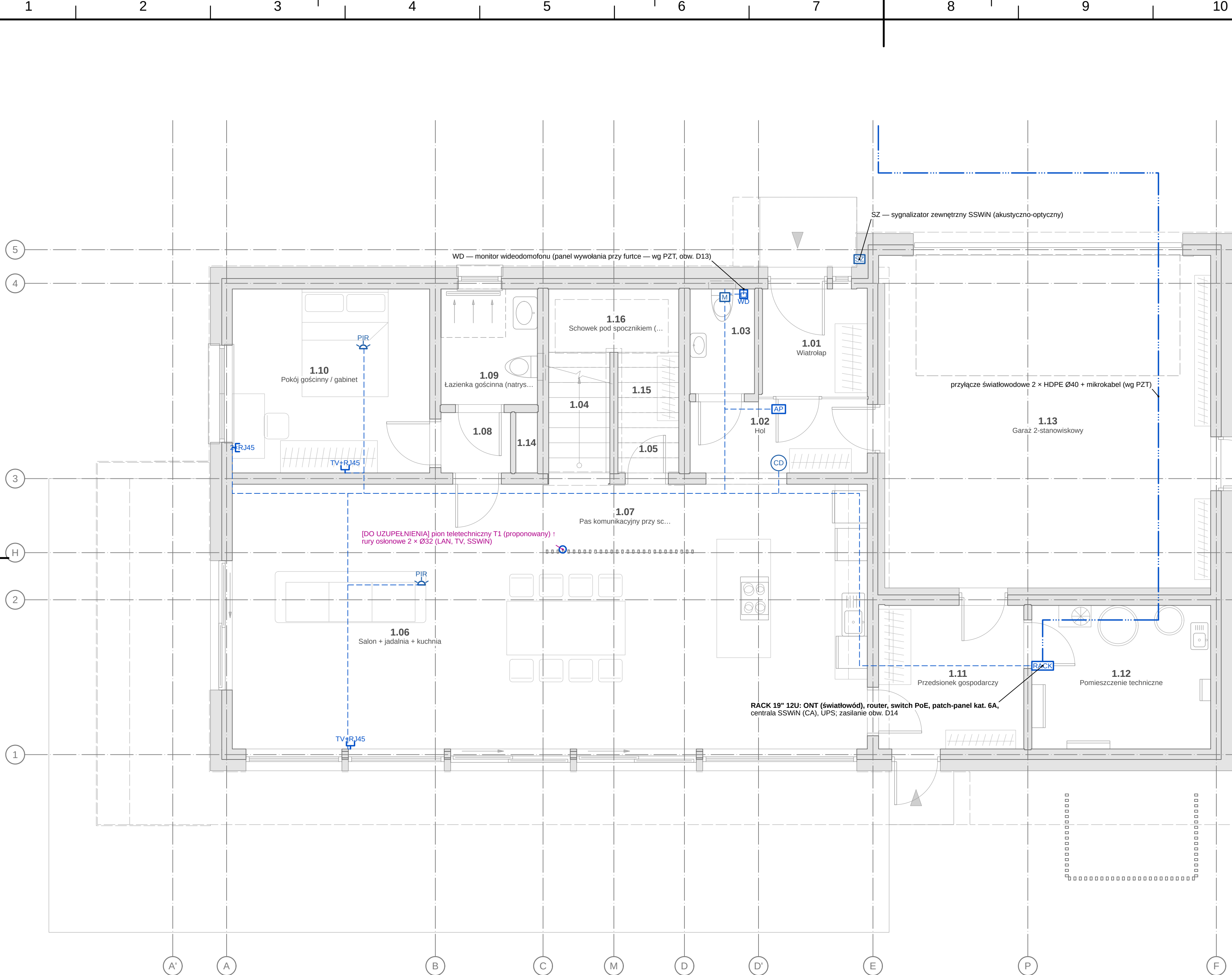
TELETECHNIKA — RZUT PARTERU 1:50
