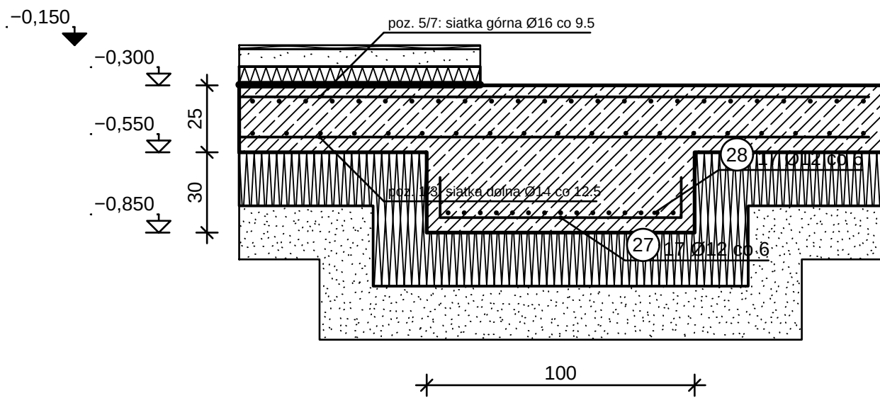
PRZEKRÓJ 3-3 — POGRUBIENIE SF1 1:20
