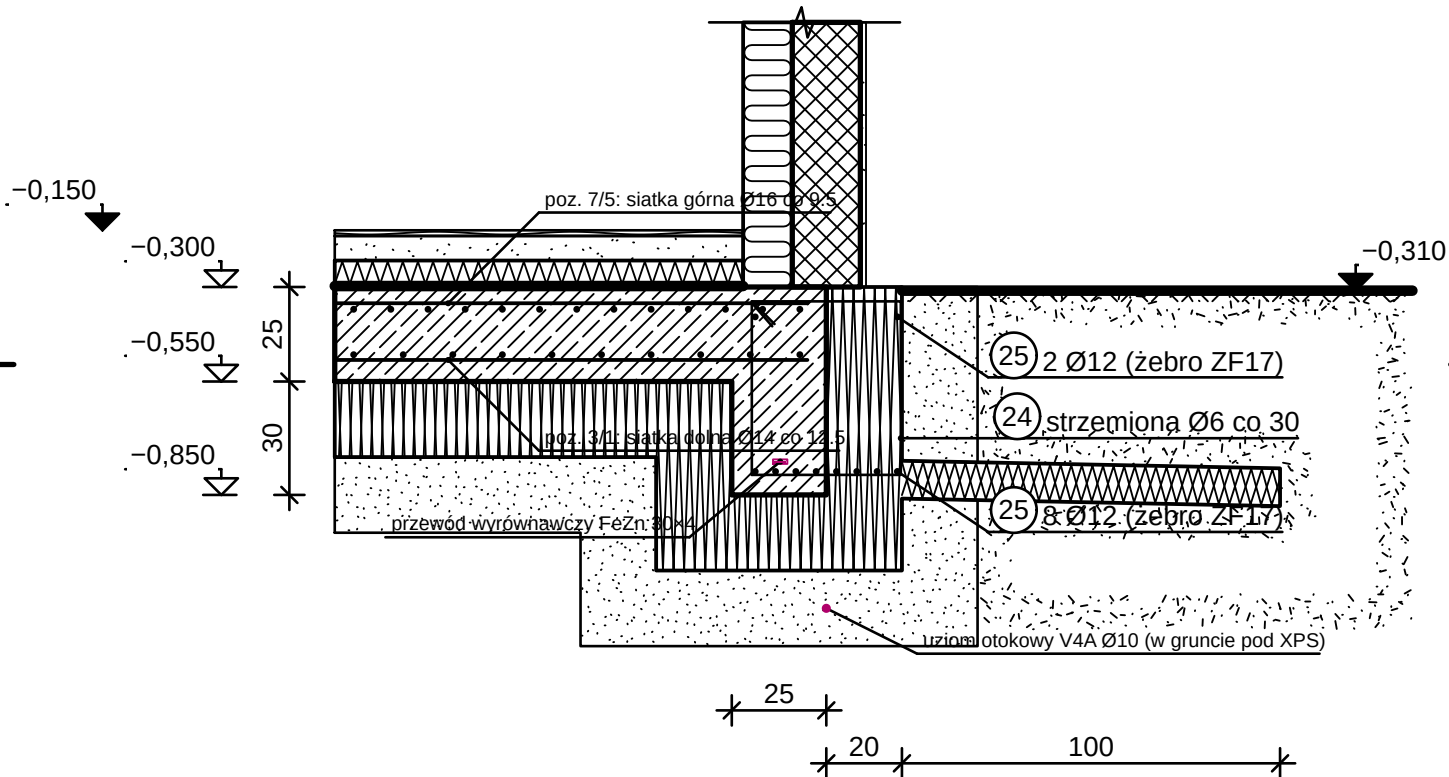
PRZEKRÓJ 2-2 — ŻEBRO ZF17 1:20
