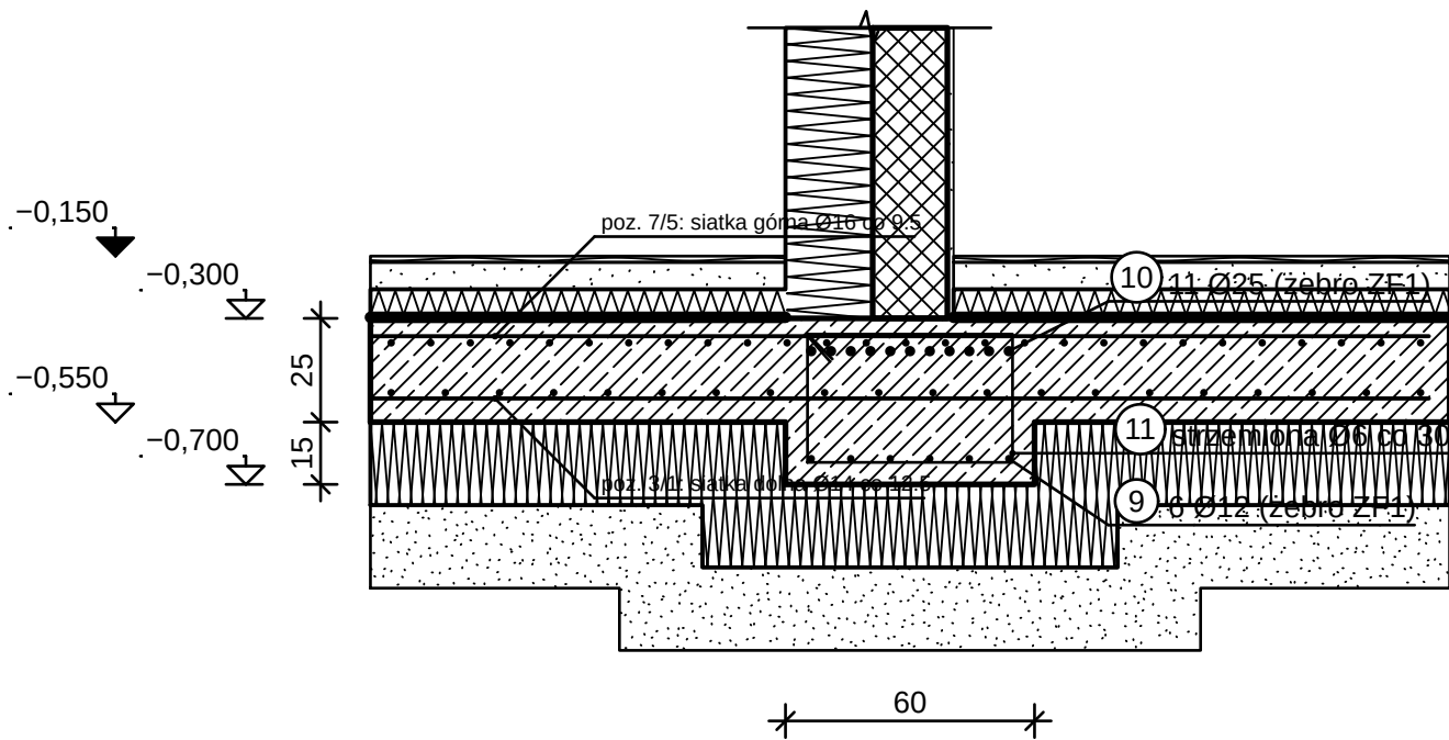
PRZEKRÓJ 1-1 — ŻEBRO ZF1 1:20
