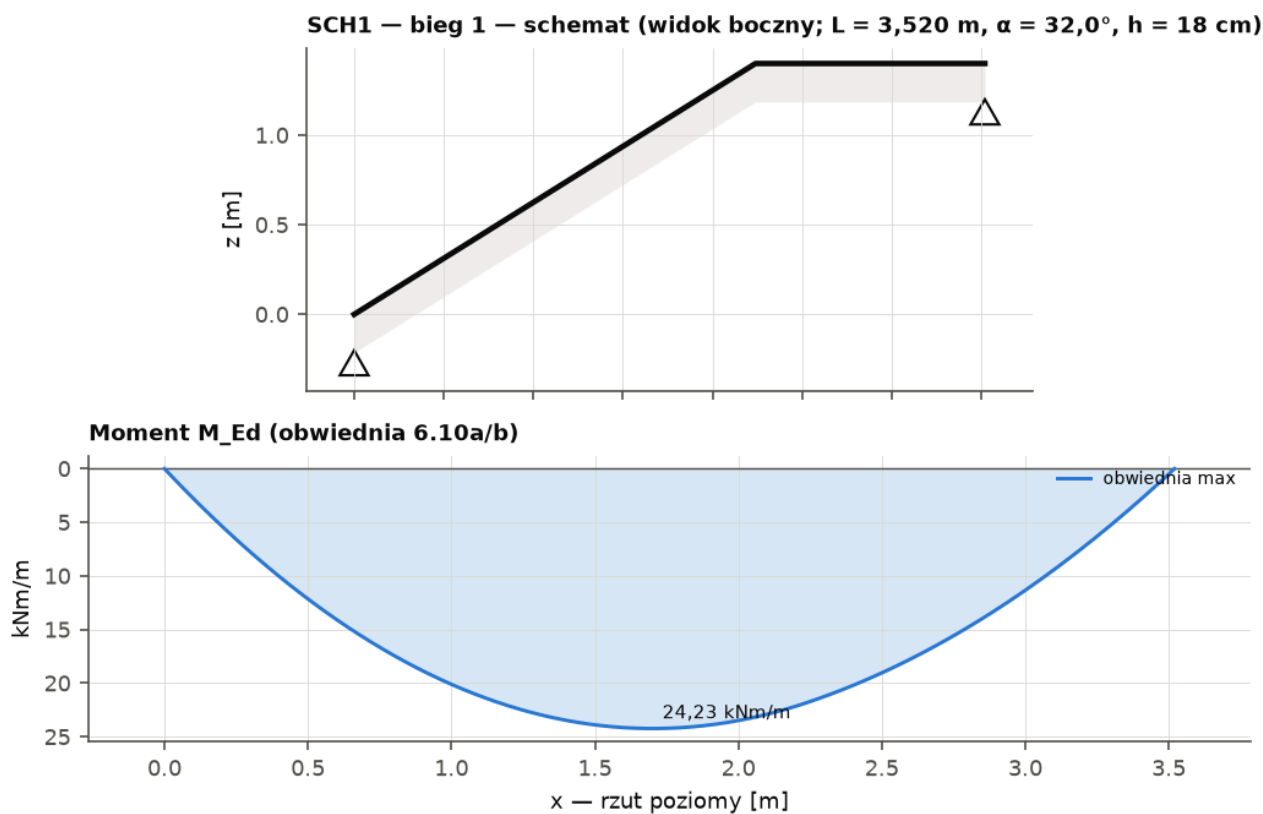
Ilustracja 28. SCH1 — bieg 1: schemat statyczny płyty schodowej i obwódca momentów zginających.
