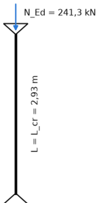
Ilustracja 66. Słup SL20: schemat statyczny (przegubowo-przesuwny, układ usztywniony).
