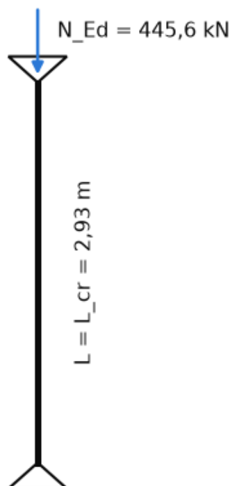
Ilustracja 58. Słup SL12: schemat statyczny (przegubowo-przesuwny, układ usztywniony).
