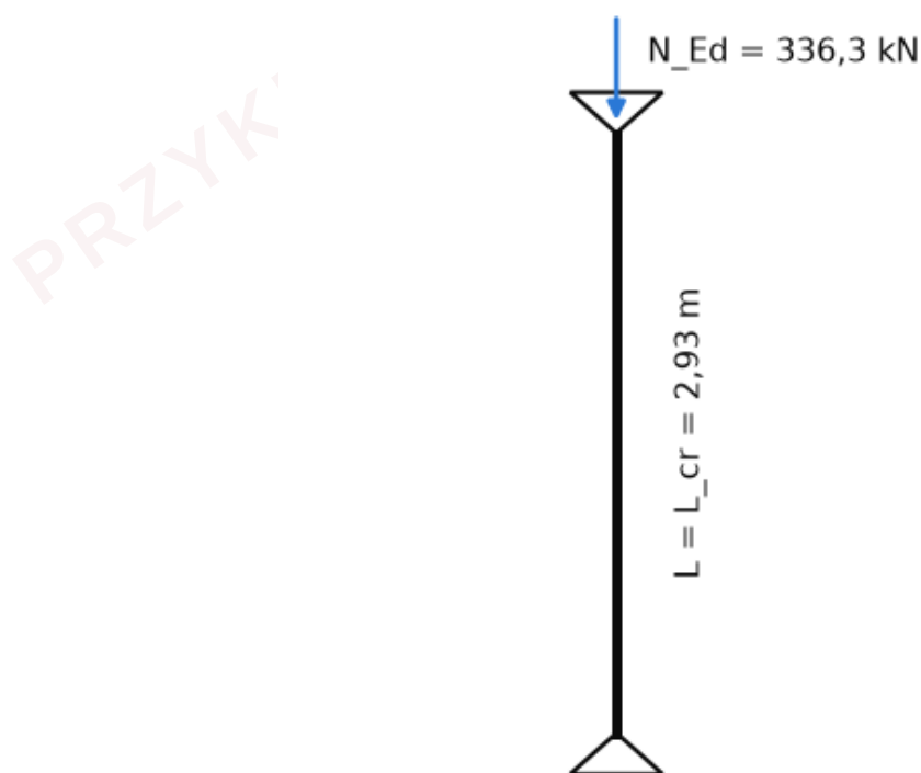
Ilustracja 61. Słup SL15: schemat statyczny (przegubowo-przesuwny, układ usztywniony).
