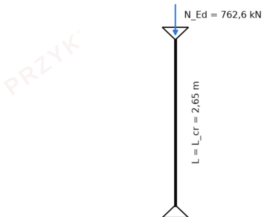
Ilustracja 65. Słup SL19: schemat statyczny (przegubowo-przesuwny, układ usztywniony).
