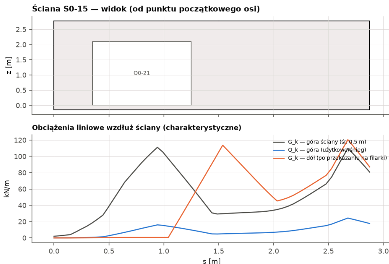
Ilustracja 93. Ściana S0-15: widok z otworami i rozkład obciążeń charakterystycznych wzdłuż osi.
