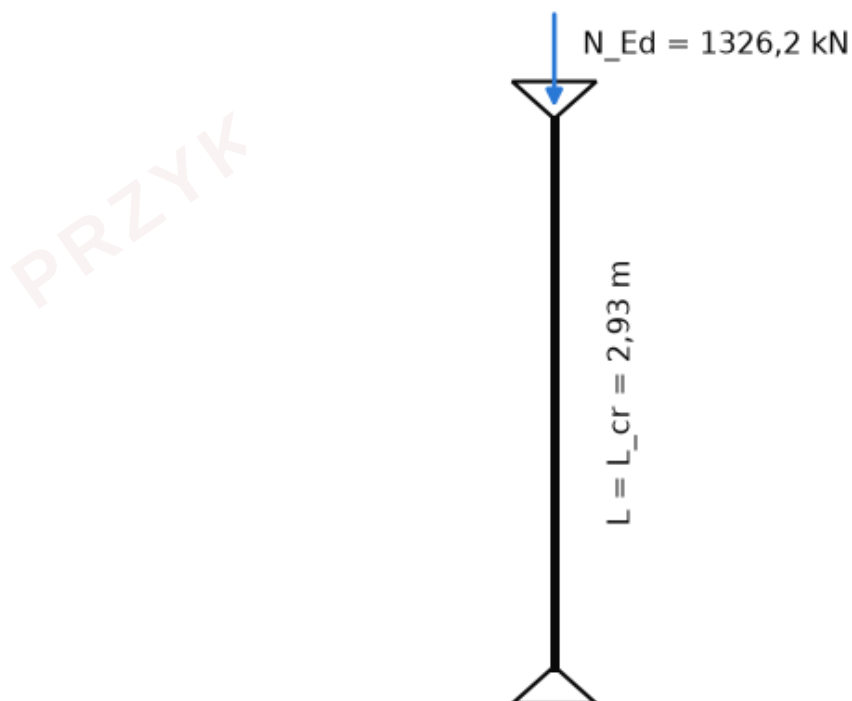
Ilustracja 59. Słup SL13: schemat statyczny (przegubowo-przesuwny, układ usztywniony).
