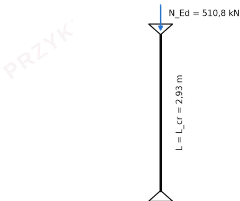
Ilustracja 57. Słup SL11: schemat statyczny (przegubowo-przesuwny, układ usztywniony).
