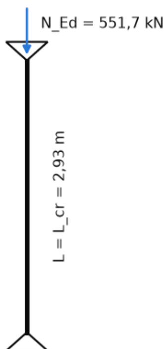
Ilustracja 56. Słup SL10: schemat statyczny (przegubowo-przesuwny, układ usztywniony).
