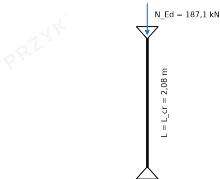
Ilustracja 67. Słup SL21: schemat statyczny (przegubowo-przesuwny, układ usztywniony).
