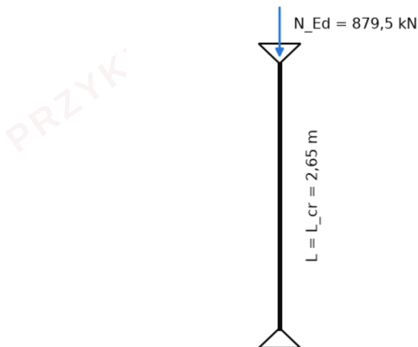
Ilustracja 63. Słup SL17: schemat statyczny (przegubowo-przesuwny, układ usztywniony).
