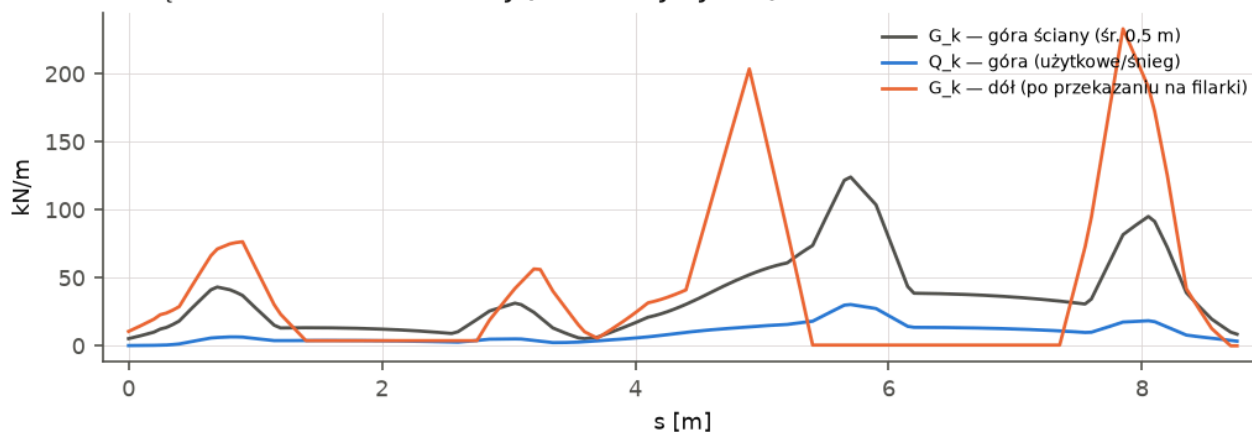
Ilustracja 88. Ściana S0-07: widok z otworami i rozkład obciążeń charakterystycznych wzdłuż osi.
