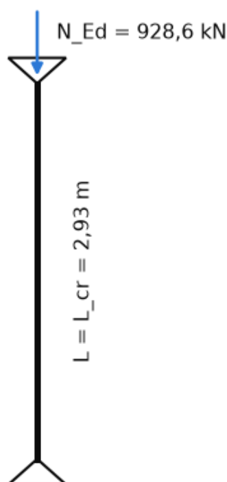
Ilustracja 60. Słup SL14: schemat statyczny (przegubowo-przesuwny, układ usztywniony).
