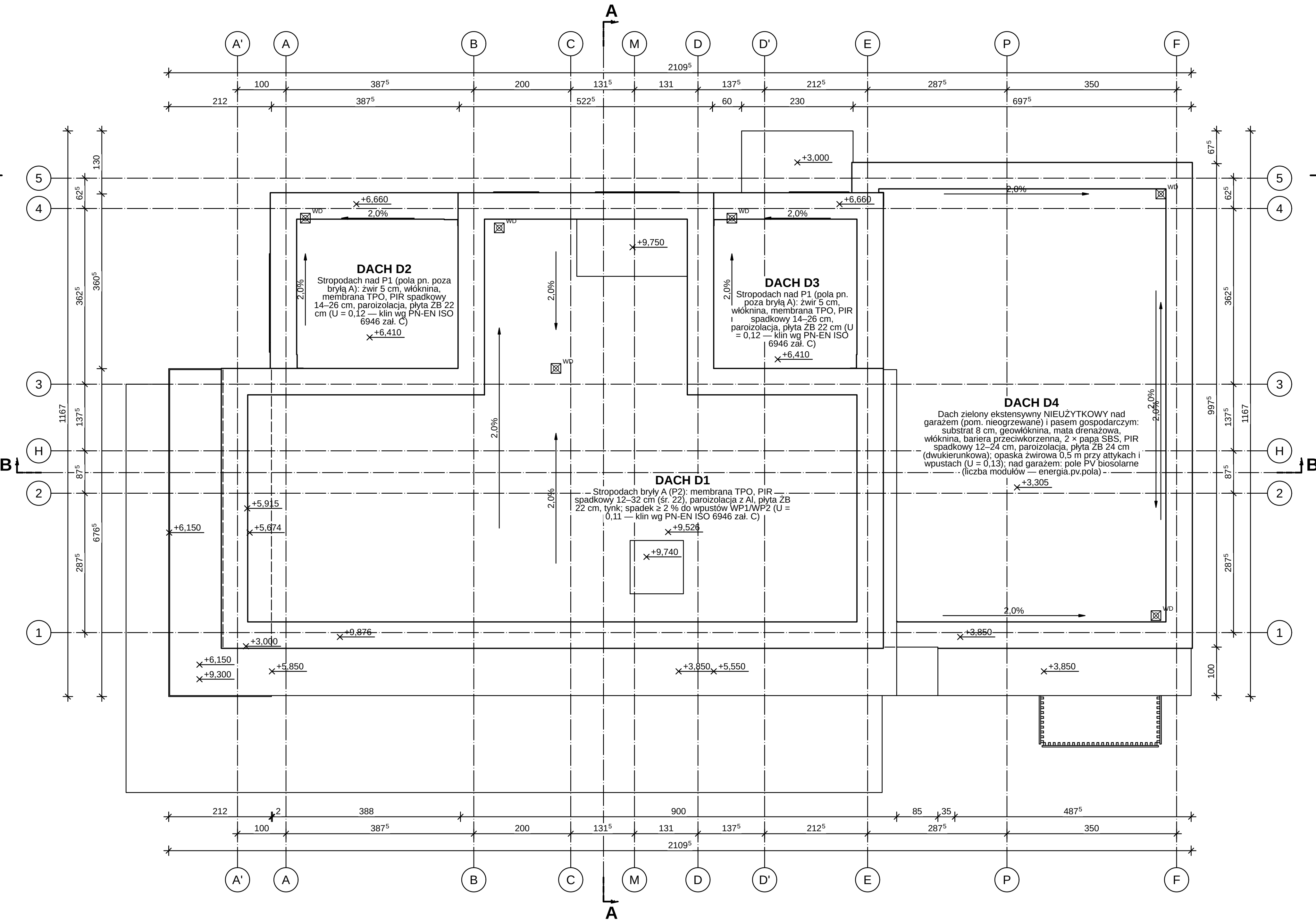
RZUT DACHU 1:50
