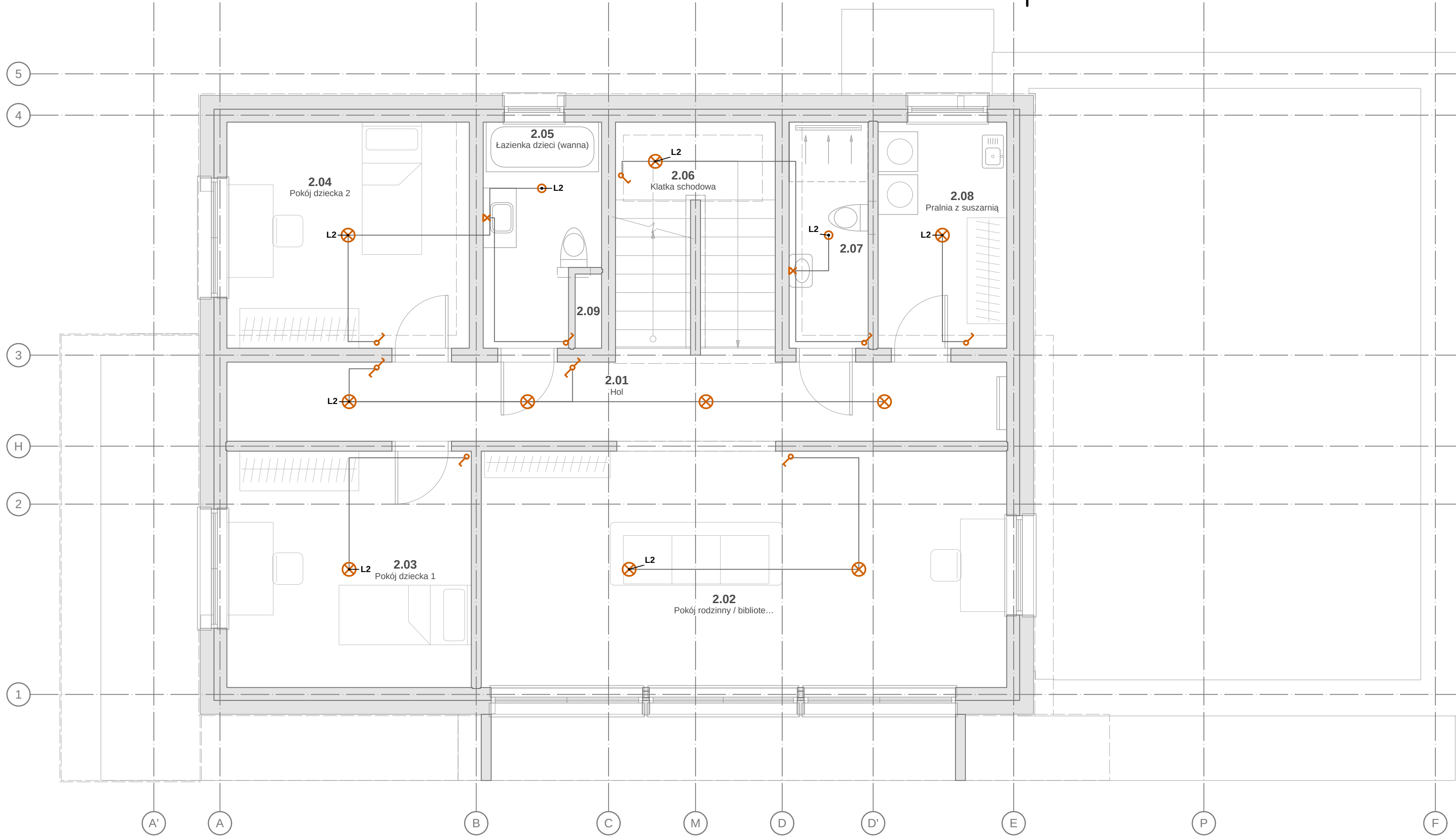
INSTALACJA OŚWIETLLENIA — RZUT I PIĘTRA 1:50
