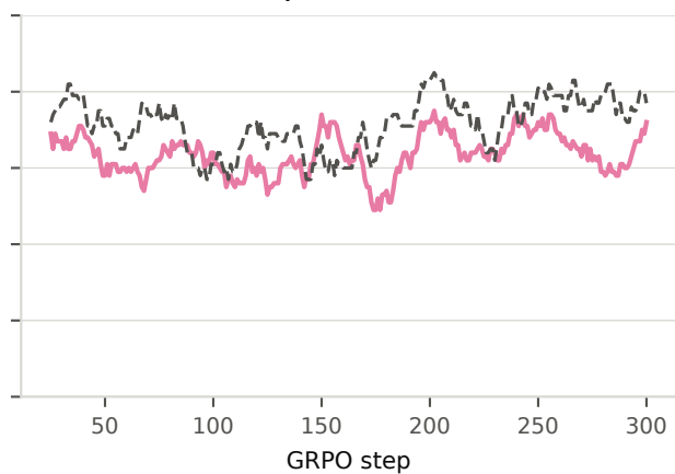
Qwen3-14B
