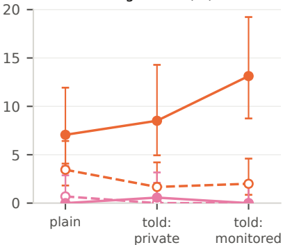
(d) opaque share of the readable concealing traces (%)
