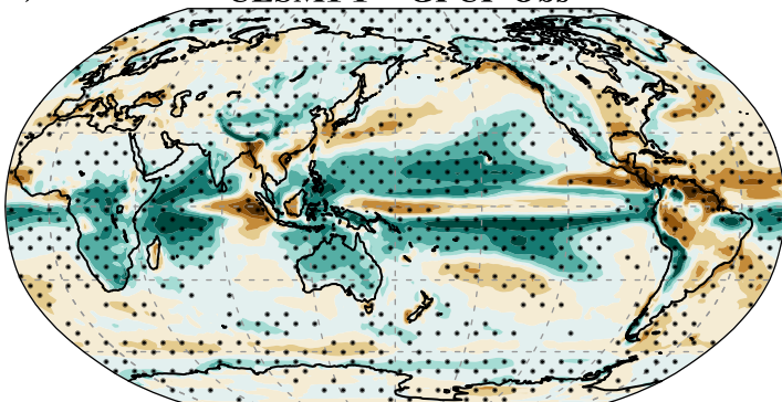
e) ANN CESM1 1° - GPCP Obs
