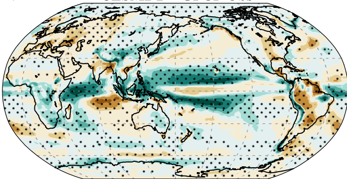
d) ANN CESM2 1° - GPCP Obs
