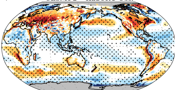
c) ANN CESM1 2° - HadCRU Obs.
