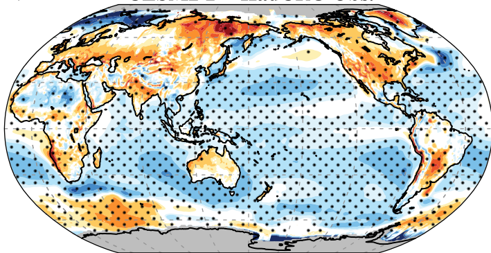
a) ANN CESM2 1° - HadCRU Obs.
