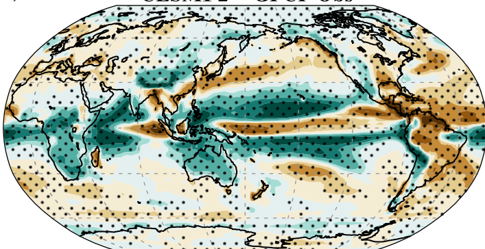
f) ANN CESM1 2° - GPCP Obs
