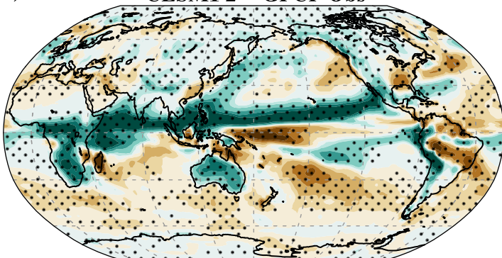
f) DJF CESM1 2° - GPCP Obs
