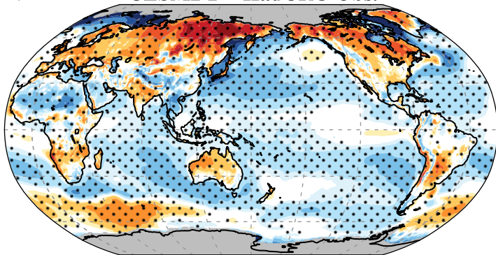
a) DJF CESM2 1° - HadCRU Obs.
