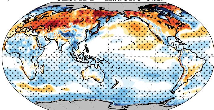
b) DJF CESM1 1° - HadCRU Obs.
