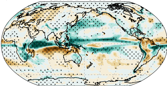
d) DJF CESM2 1° - GPCP Obs
