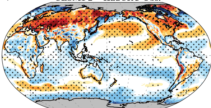
c) DJF CESM1 2° - HadCRU Obs.
