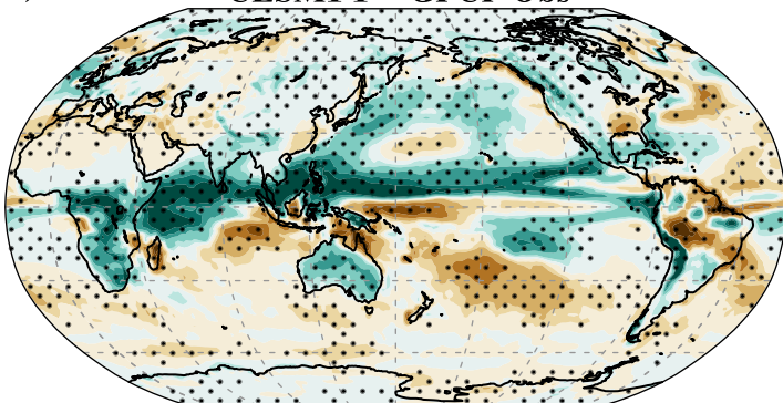
e) DJF CESM1 1° - GPCP Obs
