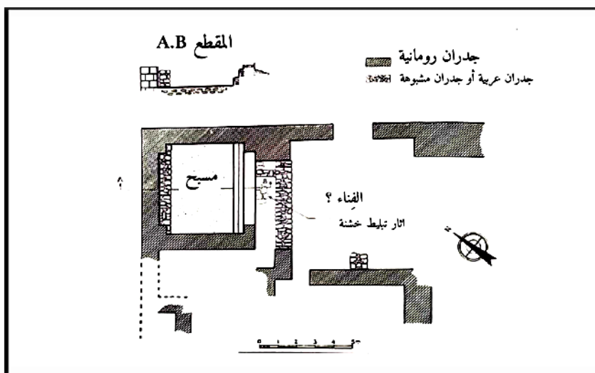
الشكل 2: يوضح مخطط المسبح، بتصريف الباحث عن: (cadenat, 1958)
