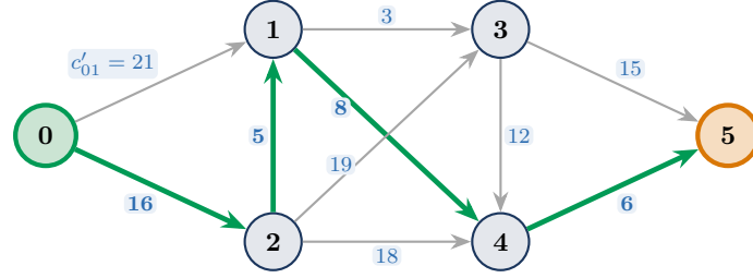
(b) Lagrangian Subproblem: Modified Costs c'_{ij} = c_{ij} + 2t_{ij}
