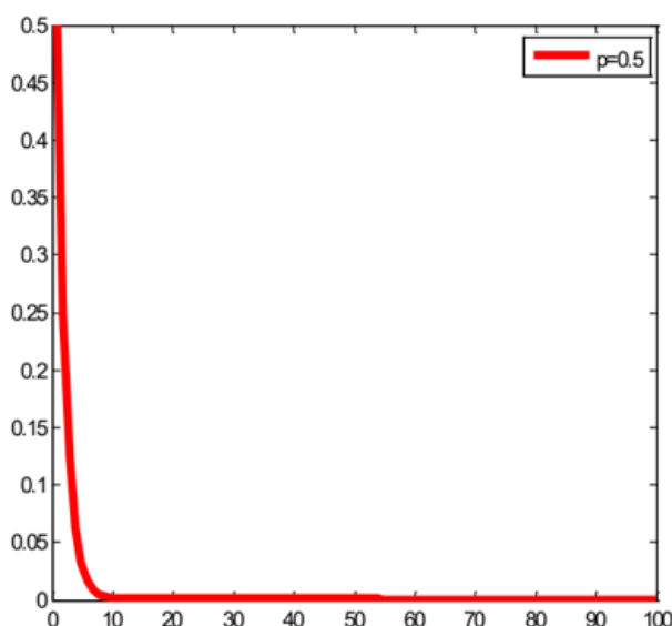
图 10: 几何分布概率质量函数 ( p = 0.5 )
