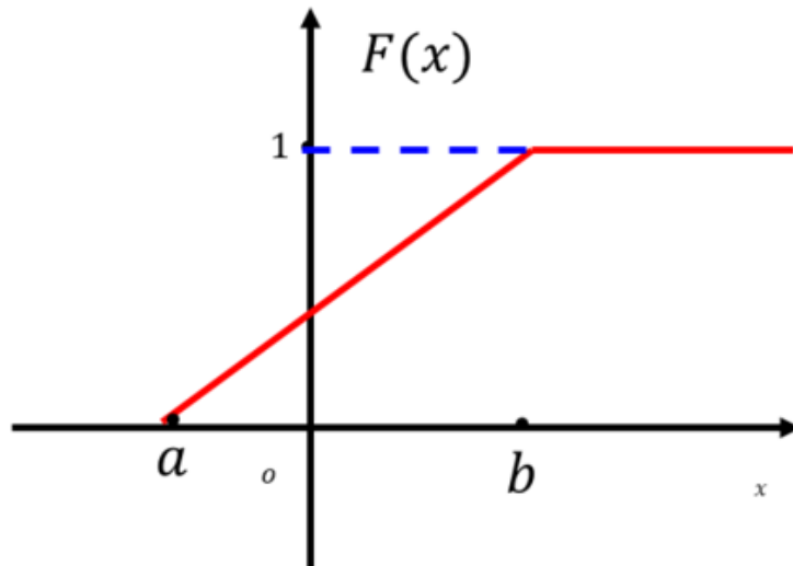
图 13: 均匀分布密度函数与分布函数
