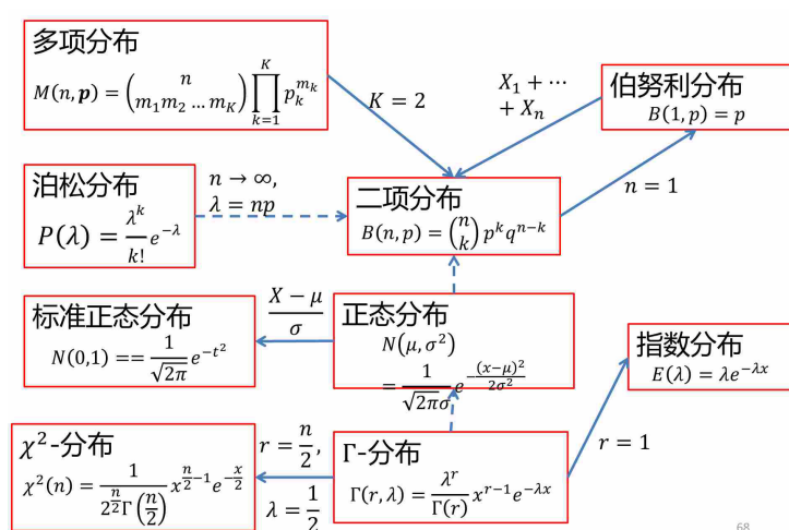
图 18: 常用概率分布及其关系总图
