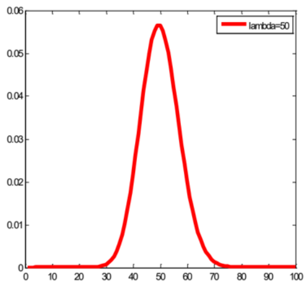
图 8: Poisson 分布概率质量函数 ( \lambda = 50 )
