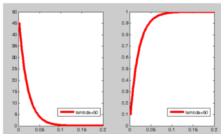
图 14: 指数分布密度函数与分布函数
