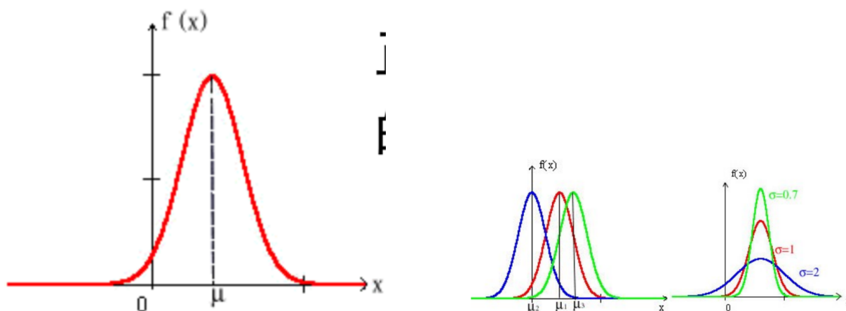
图 16: 正态分布密度曲线对比（左：不同 \mu ；右：不同 \sigma ）
