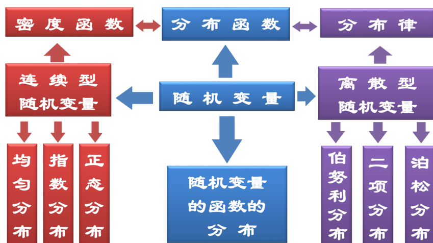
图 6: 第二章知识结构图
