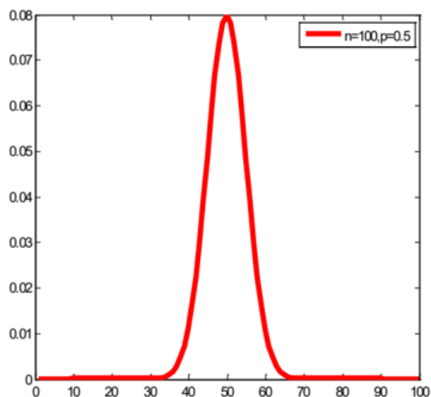
图 7: 二项分布概率质量函数 ( n = 100, p = 0.5 )
