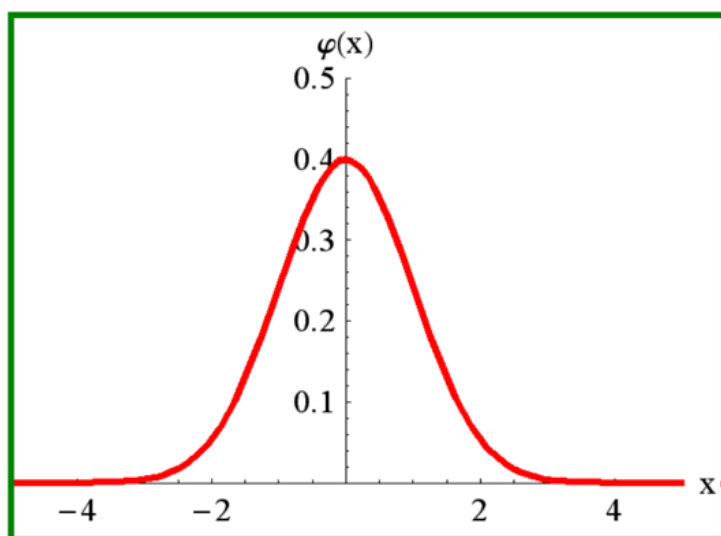
图 17: 标准正态分布密度函数 \varphi(x) 与分布函数 \Phi(x)
