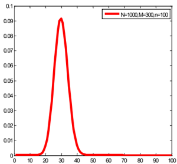
图 11: 超几何分布概率质量函数
