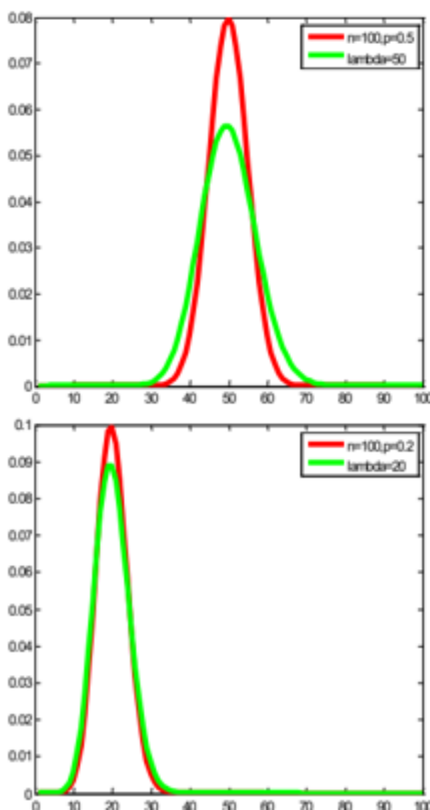
图 9: Poisson 定理近似效果图
