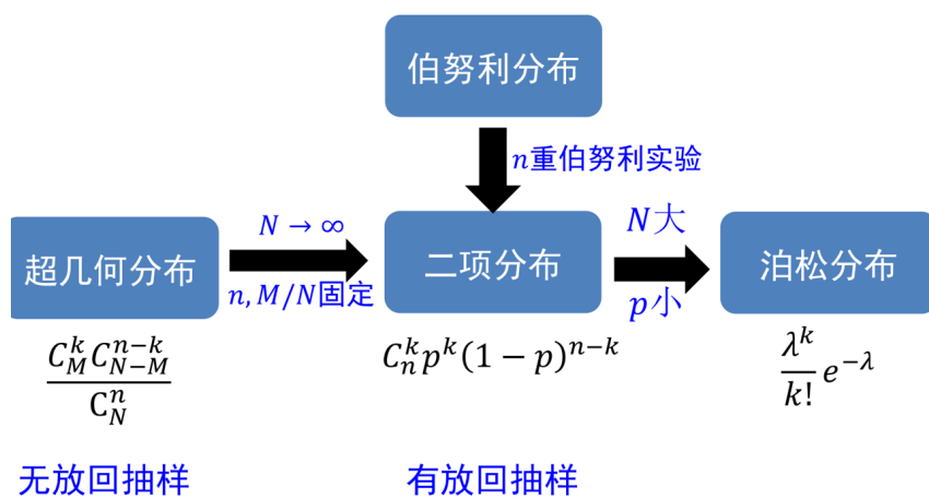
图 12: 常用离散型分布关系图
