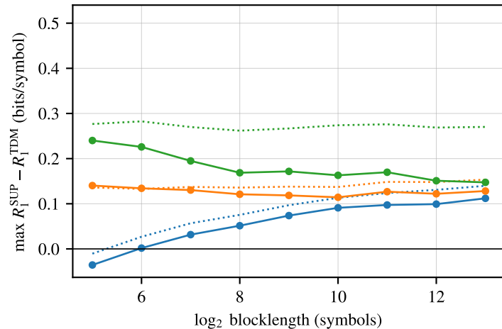
8PSK
