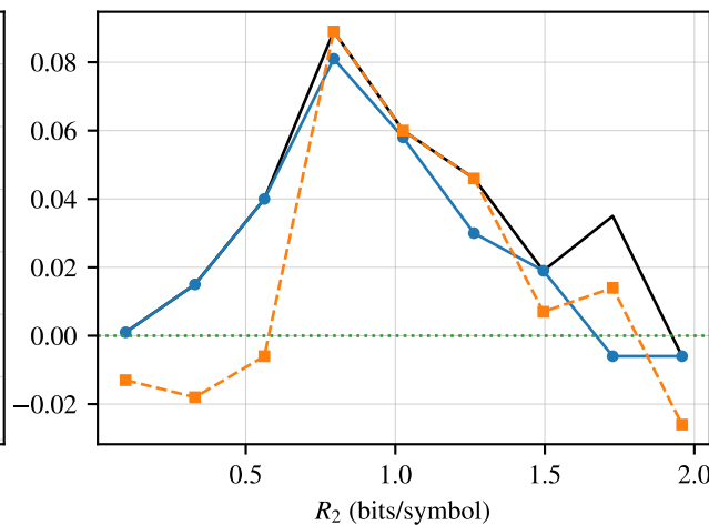
8QAM 13 / 8 dB, n = 2048
