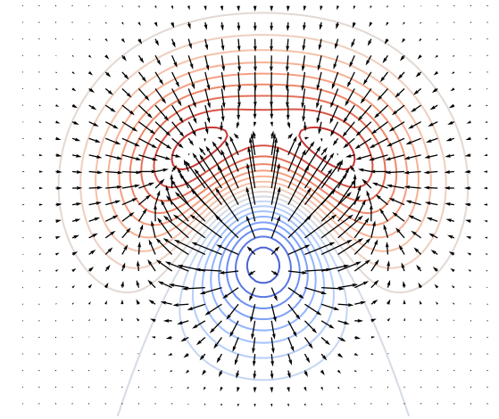
FIGURE 8.3 – Champ de vecteurs de \nabla f , et lignes de niveau de f .
