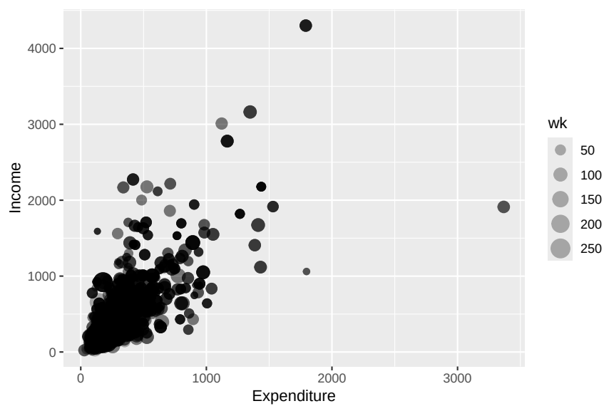
Figure 3.7: Diagrama de dispersión entre ingreso y gasto de los hogares
