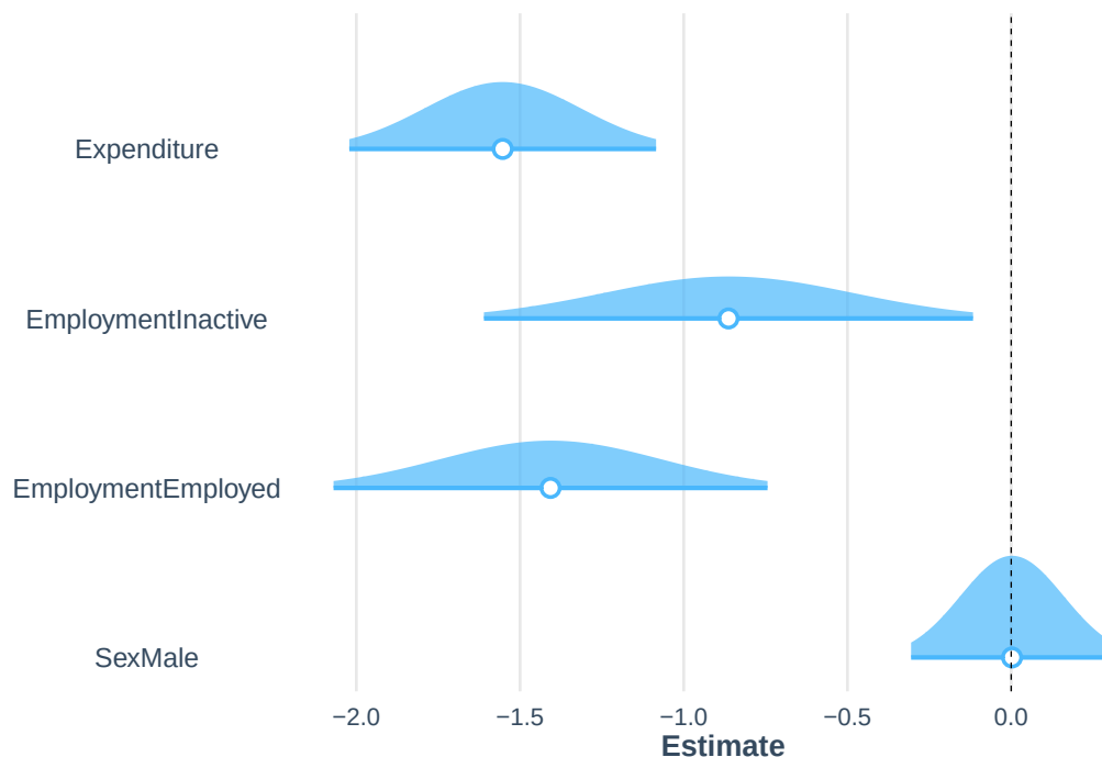
Figure 6.1: Distribución de los parámetros del modelo logístico base
