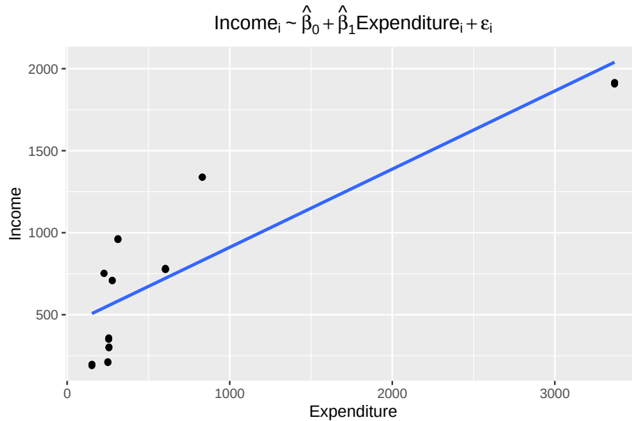
Figure 7.1: Modelo de regresión lineal simple para el ingreso en función del gasto (sin considerar estratos)
