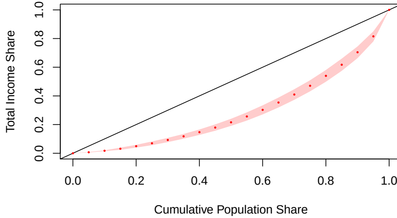
Figure 3.1: Curva de Lorenz estimada para el ingreso de los hogares
