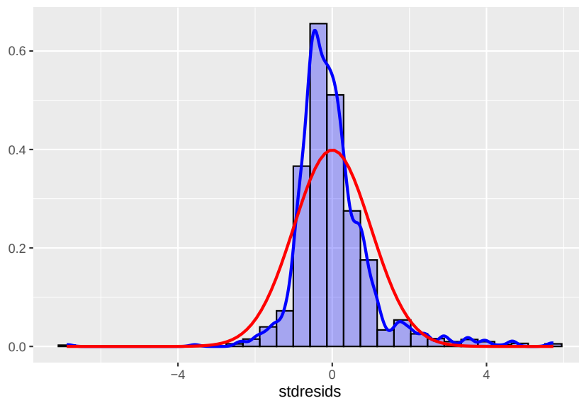
Figure 5.2: Histograma de residuales estandarizados con curva de densidad estimada y distribución normal teórica
