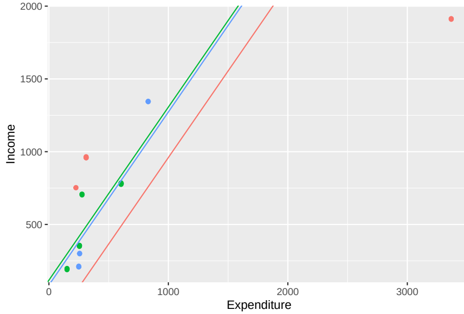
Figure 7.5: Rectas de regresión estimadas por estrato: modelo con intercepto aleatorio
