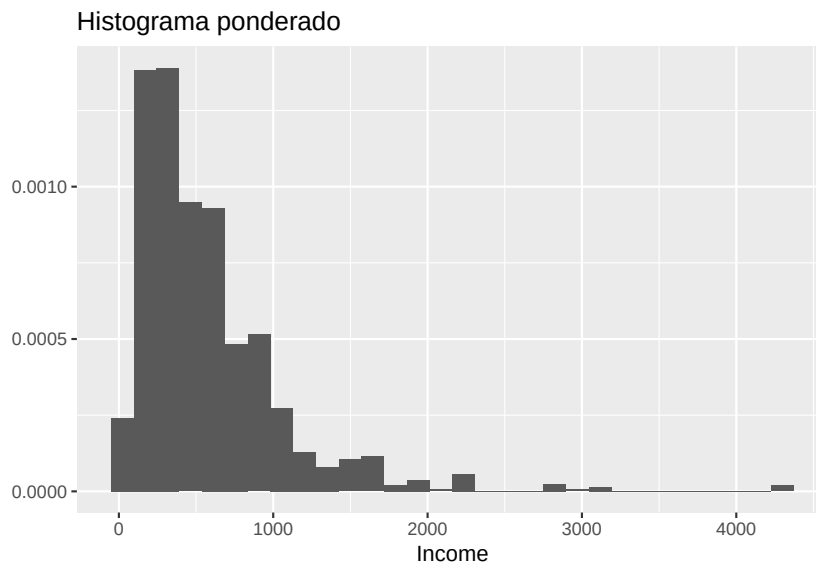
Figure 3.2: Histograma ponderado del ingreso de los hogares
