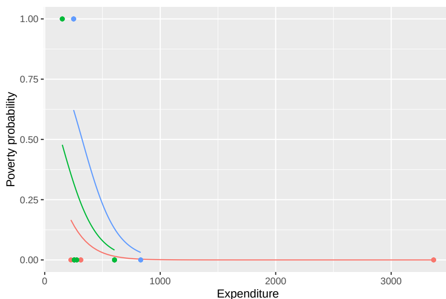
Figure 7.8: Curvas de probabilidad predichas por estrato: modelo logístico con intercepto aleatorio
