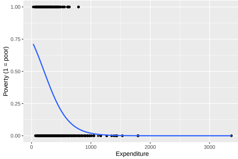
Figure 7.7: Relación entre gasto y condición de pobreza con curva logística ajustada
