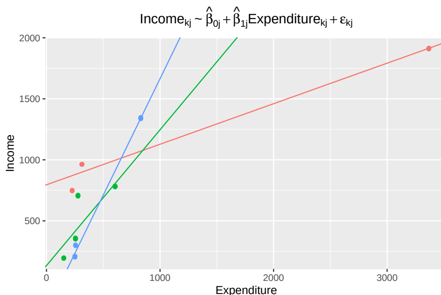
Figure 7.4: Modelo con intercepto y pendiente específicos por estrato (ajuste independiente)
