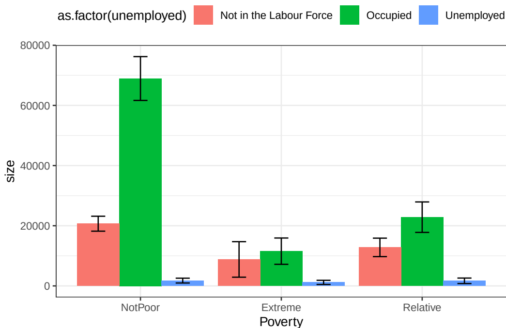
Figure 4.3: Gráfico de barras del tamaño poblacional por estado de ocupación y pobreza
