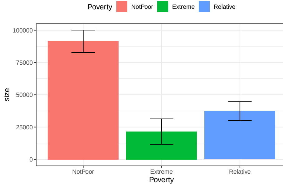
Figure 4.2: Gráfico de barras del tamaño poblacional por condición de pobreza
