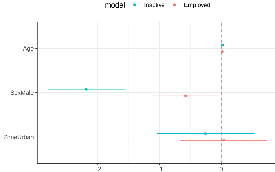
Figure 6.3: Intervalos de confianza para los coeficientes del modelo multinomial
