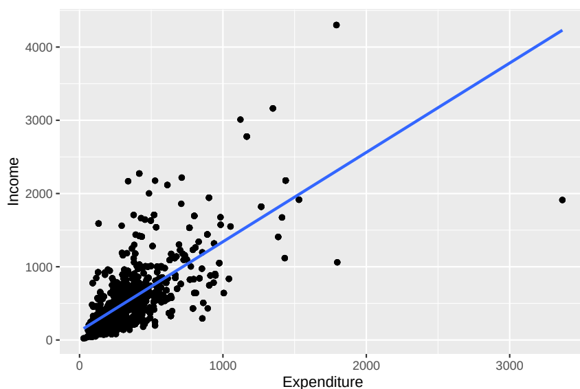
Figure 5.1: Diagrama de dispersión entre gasto e ingreso en la muestra (sin ponderar)
