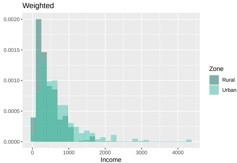
Figure 3.3: Histograma ponderado del ingreso por zona geográfica
