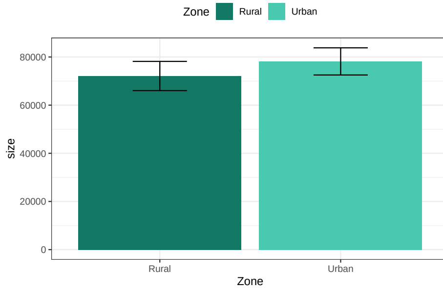
Figure 4.1: Gráfico de barras del tamaño poblacional por zona geográfica
