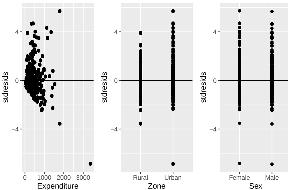
Figure 5.3: Gráficos de residuales estandarizados frente a cada covariable del modelo
