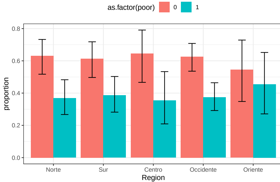
Figure 4.5: Proporción de hombres en condición de pobreza por región
