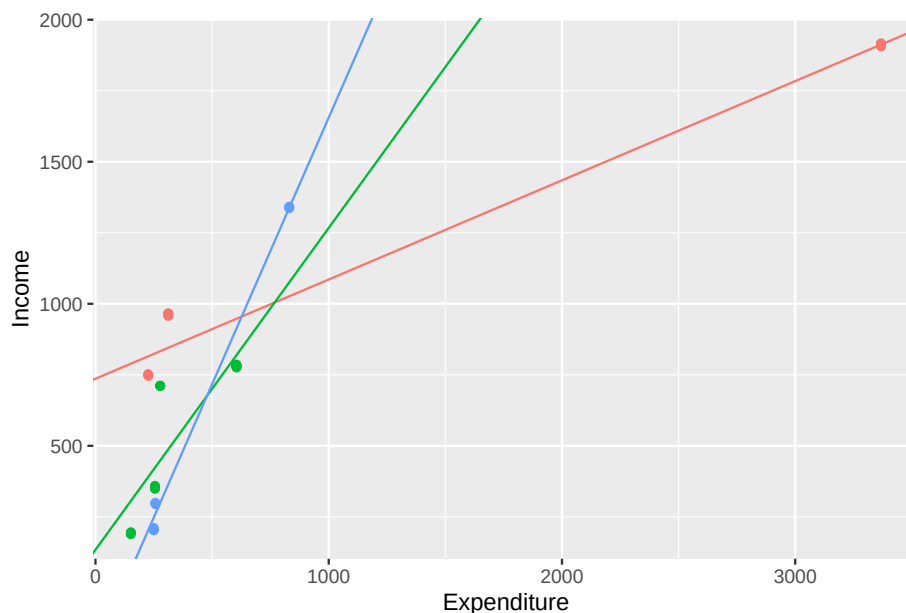
Figure 7.6: Rectas de regresión estimadas por estrato: modelo con intercepto y pendiente aleatoria
