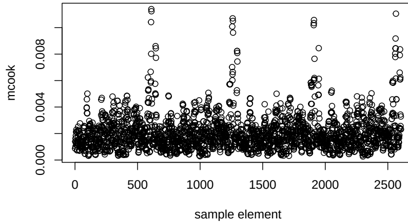
Figure 5.4: Distancia de Cook para cada observación de la muestra
