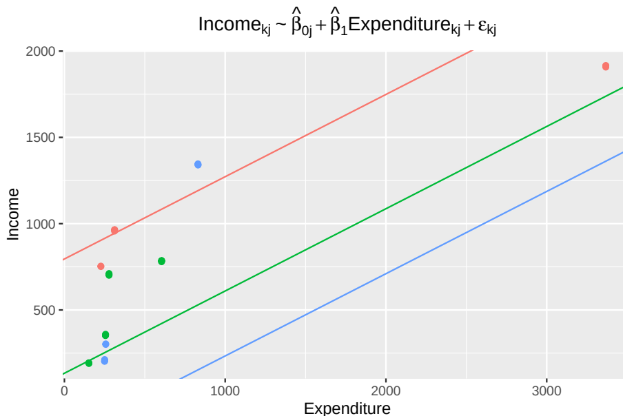
Figure 7.2: Modelo con intercepto específico por estrato y pendiente común
