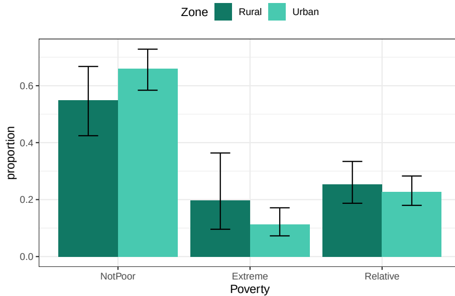
Figure 4.4: Proporción de hombres en condición de pobreza por zona geográfica
