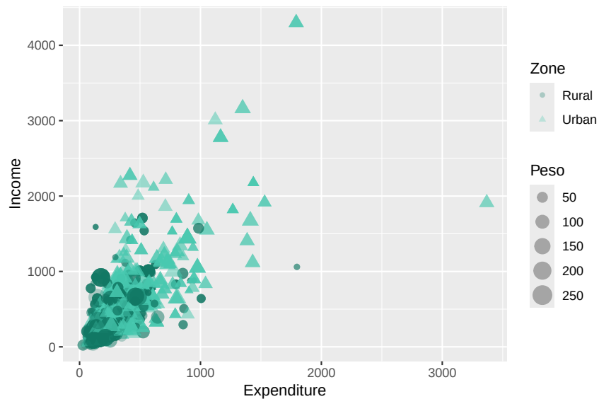
Figure 3.8: Diagrama de dispersión entre ingreso y gasto por zona geográfica
