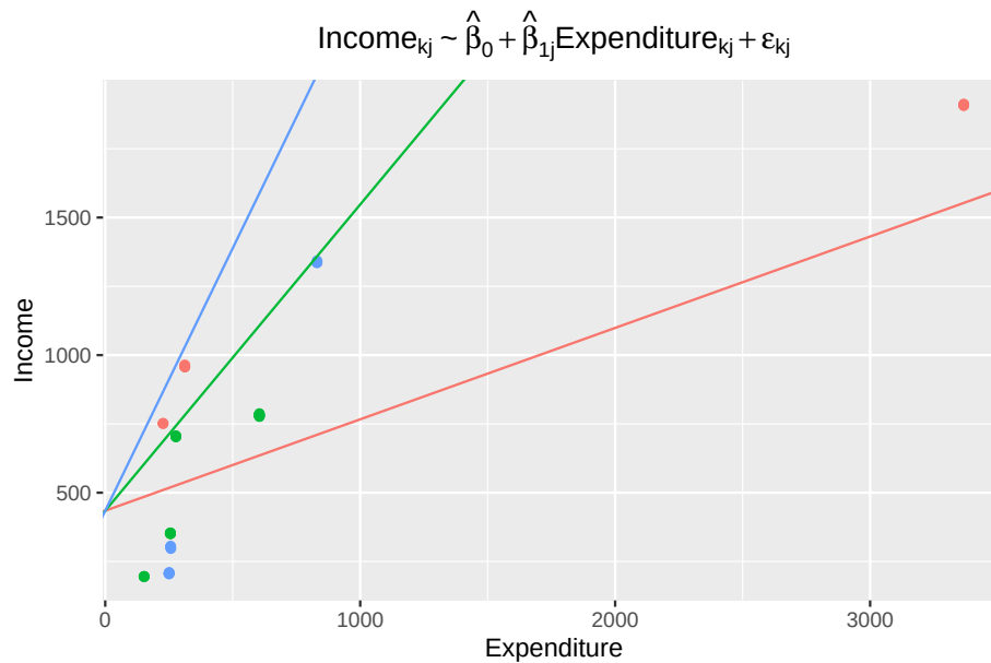
Figure 7.3: Modelo con pendiente específica por estrato e intercepto común
