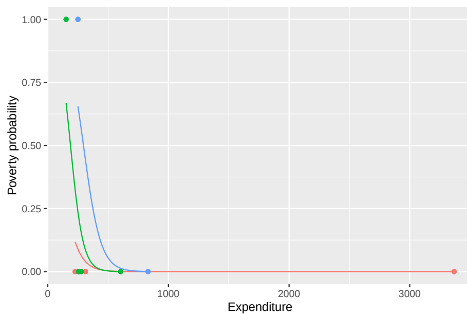
Figure 7.9: Curvas de probabilidad predichas por estrato: modelo logístico con intercepto y pendiente aleatoria
