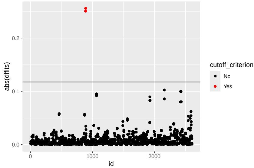
Figure 5.6: Valores DfFits: observaciones influyentes sobre el ajuste global señaladas en rojo
