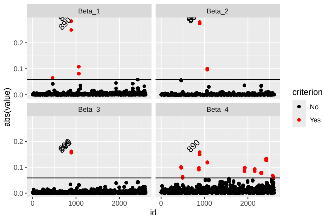
Figure 5.5: Valores DfBetas por parámetro: observaciones influyentes señaladas en rojo
