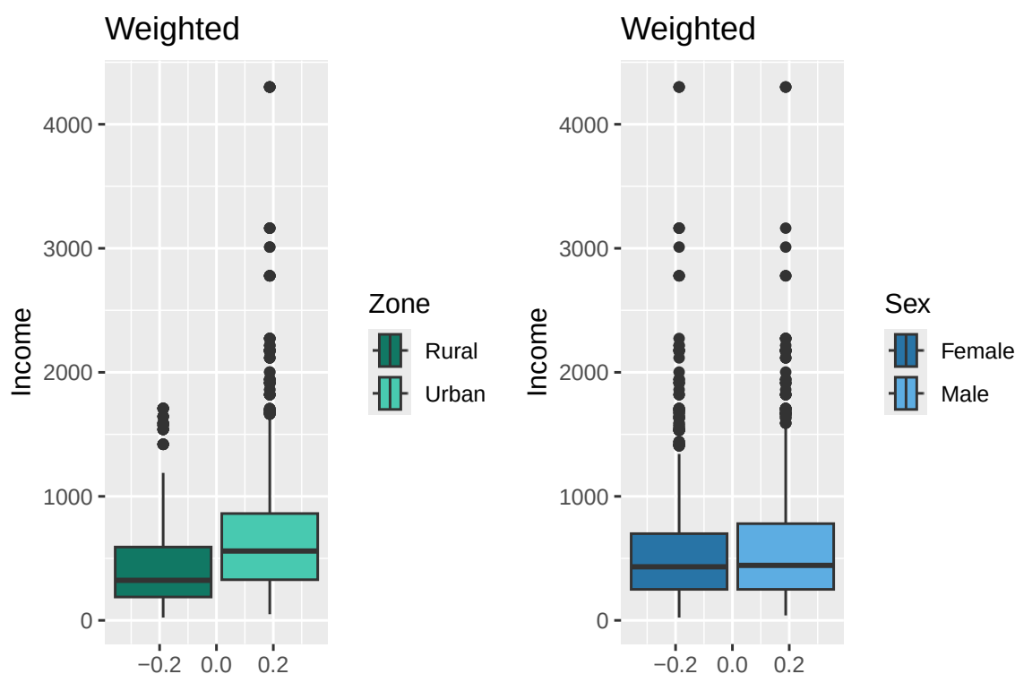
Figure 3.5: Boxplots ponderados del ingreso por zona y sexo
