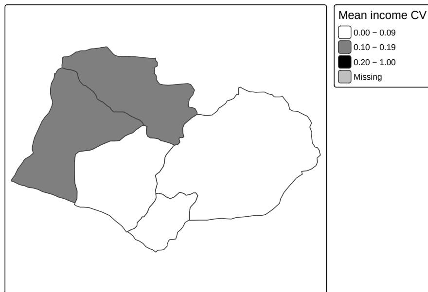
Figure 4.8: Coeficiente de variación del ingreso medio por región
