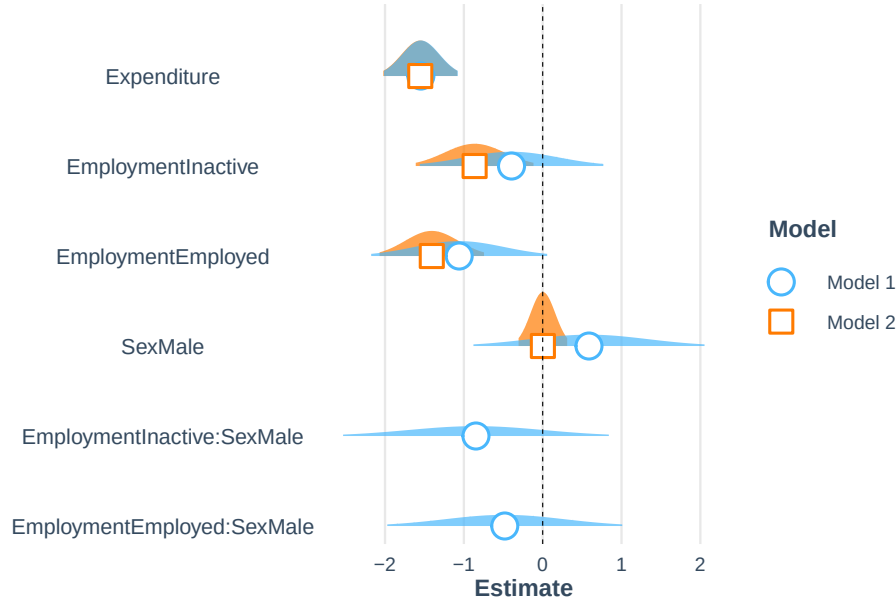
Figure 6.2: Comparación de los parámetros del modelo logístico con y sin interacciones
