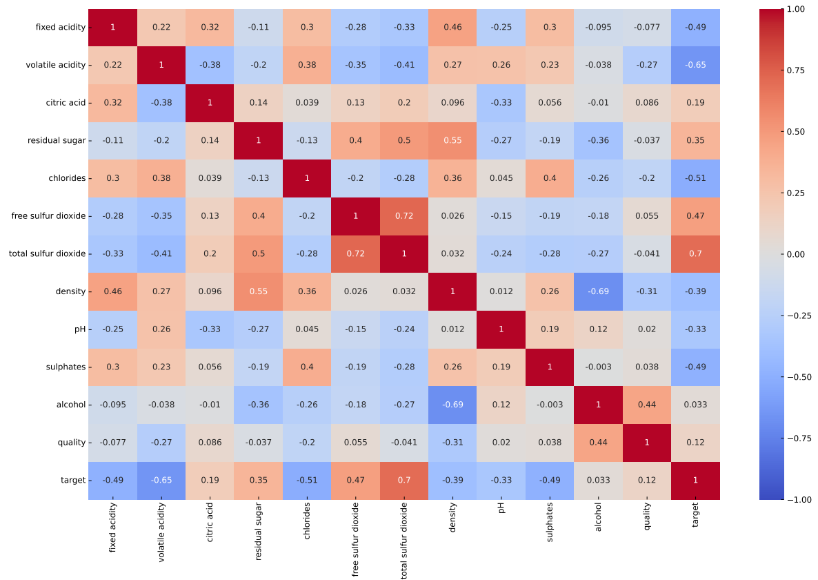
Рисунок 2.1 – Корреляционная матрица признаков
