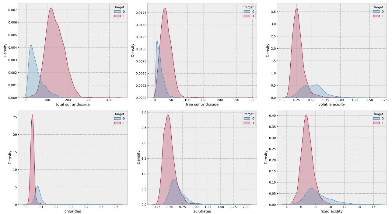
Рисунок 2.2 – Распределения признаков по классам (KDE)
