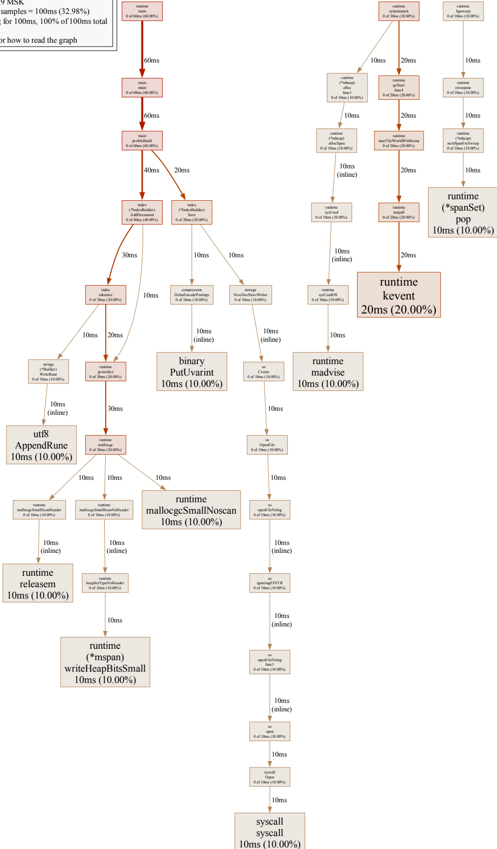
Рисунок 3.6 – CPU-профиль построения индекса
