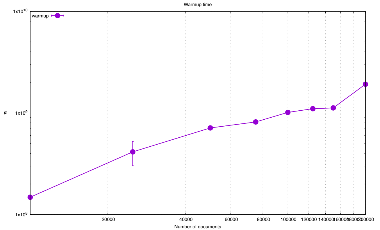
Рисунок 3.2 – Время первого запроса после загрузки индекса (warmup)
