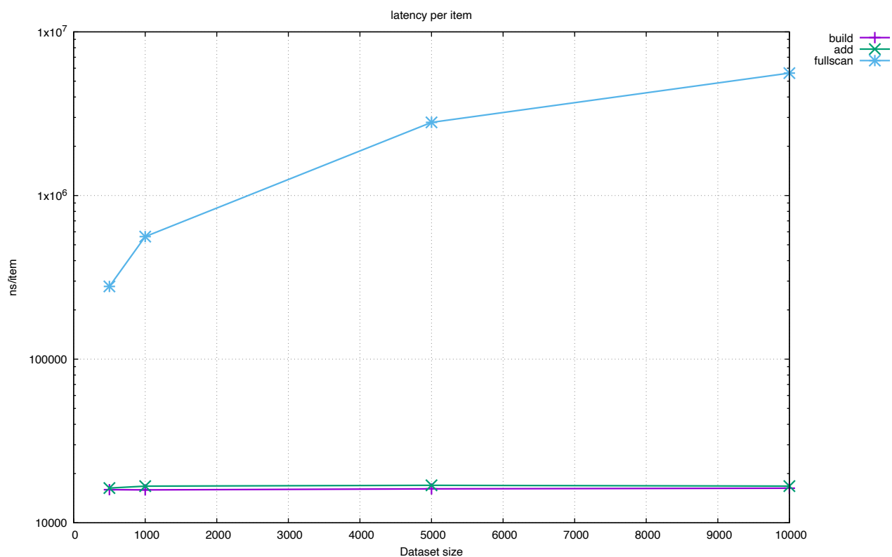
Рисунок 3.7 – Задержка операций min hash на элемент
