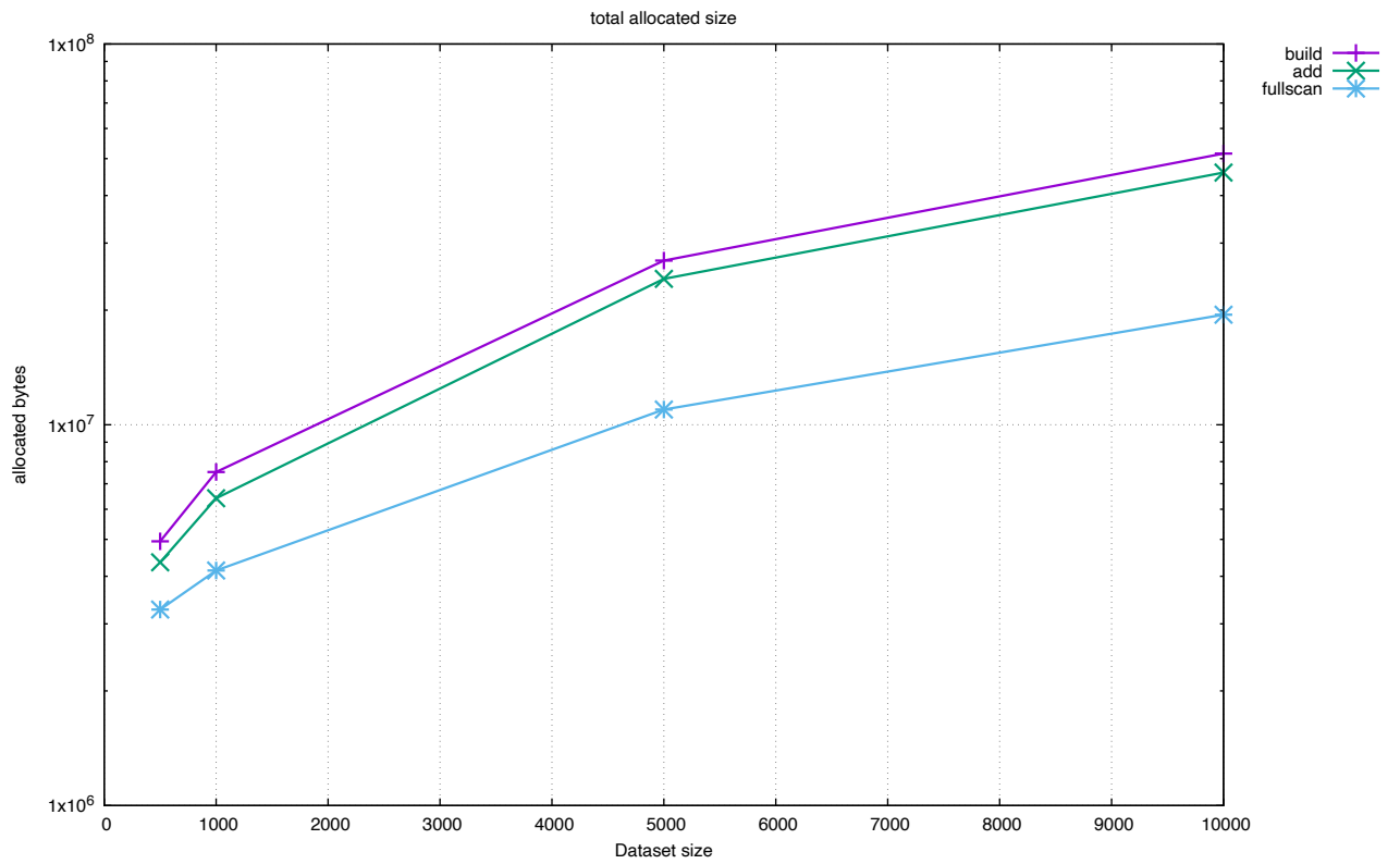
Рисунок 3.9 – Суммарный размер аллокаций для min hash
