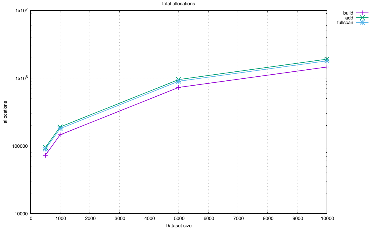
Рисунок 3.10 – Общее число аллокаций для min hash
