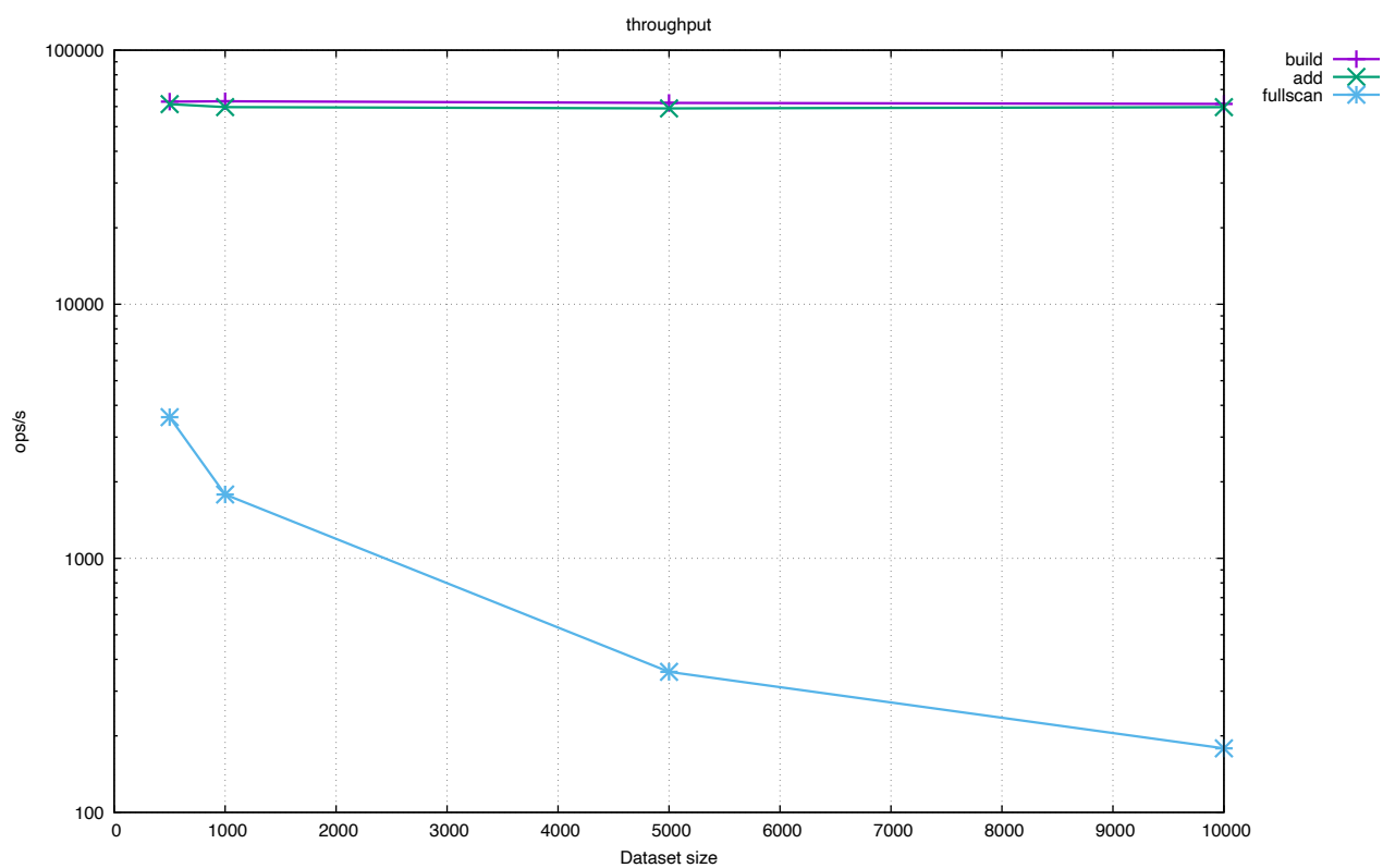
Рисунок 3.8 – Пропускная способность операций min hash
