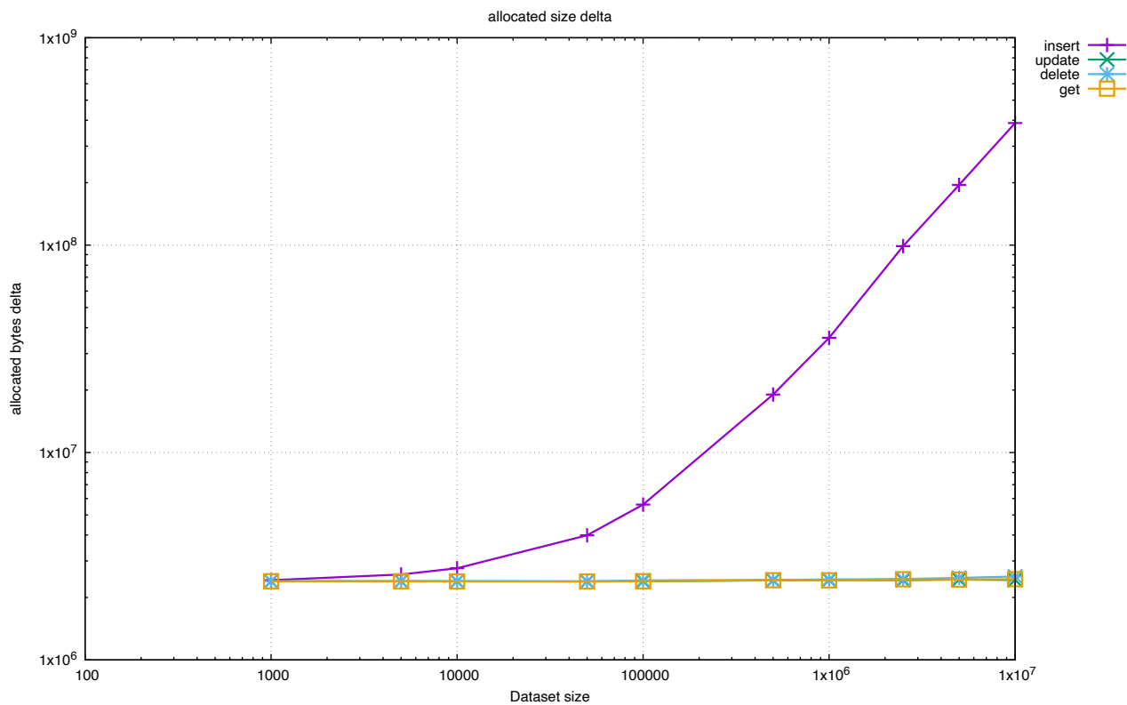
Рисунок 3.5 – Делта аллокаций для extendible hashing
