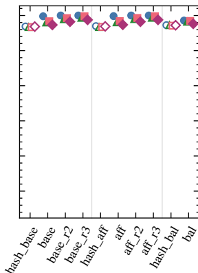
ж) частые тройки, n = 2000
