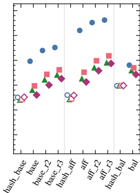
е) частые пары, n = 2000
