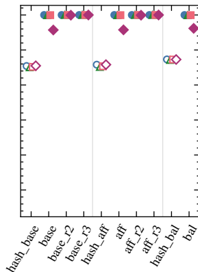
г) связанные пары, n = 2000
