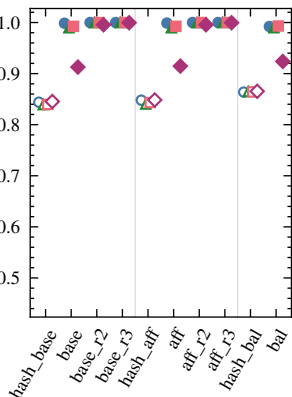
д) связанные тройки, n = 2000
