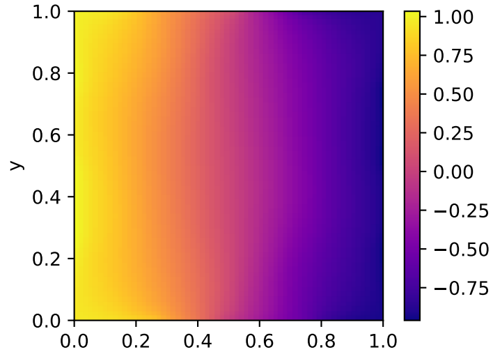
NN u(x,y)
