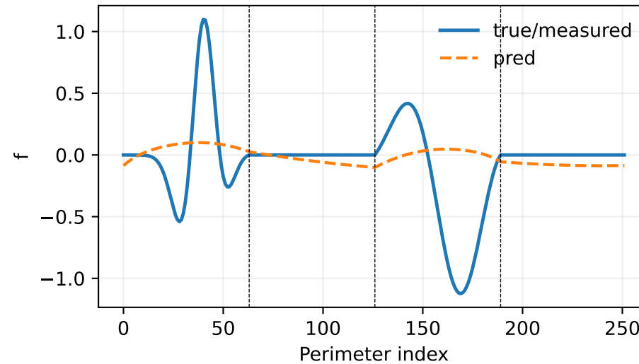
Dirichlet f_k (k=0)
