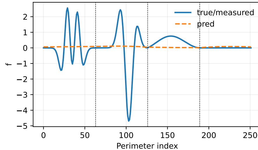
Dirichlet f_k ( k=20 )
