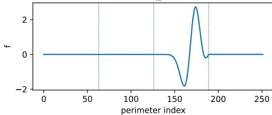
Dirichlet f_k (k=0)
