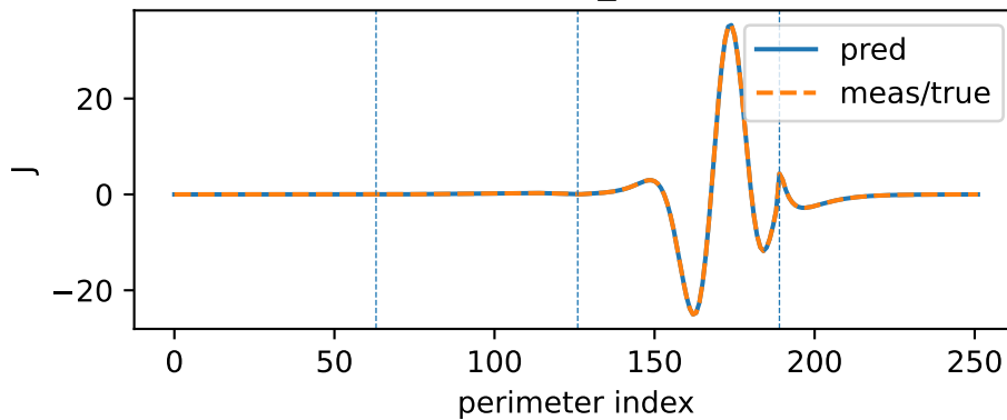
Neumann J_k (k=0)
