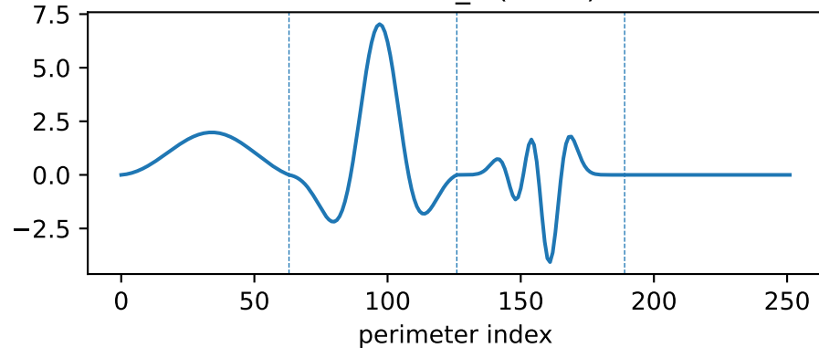
Dirichlet f_k (k=10)
