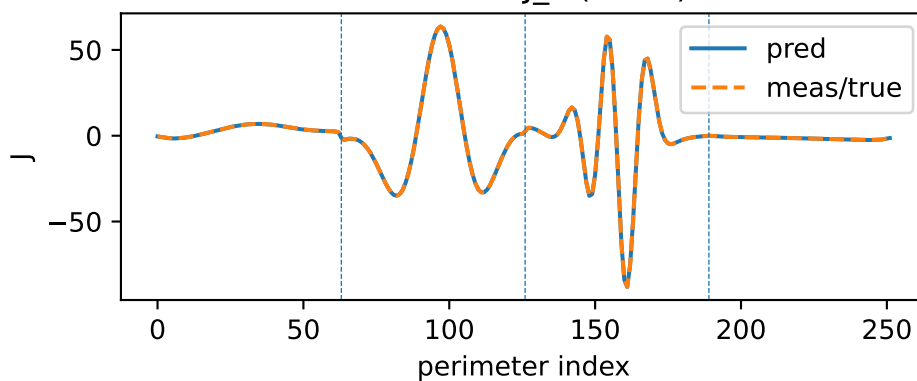
Neumann J_k (k=10)
