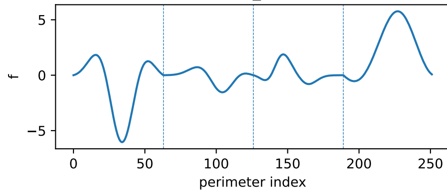
Dirichlet f_k (k=30)
