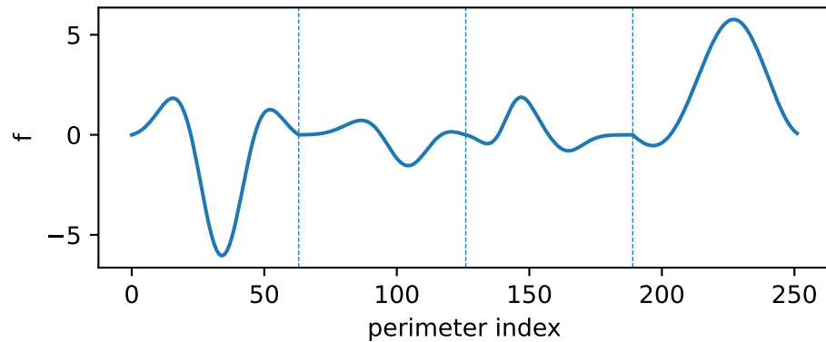
Dirichlet f_k (k=30)
