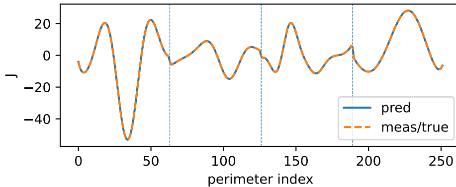
Neumann J_k (k=30)
