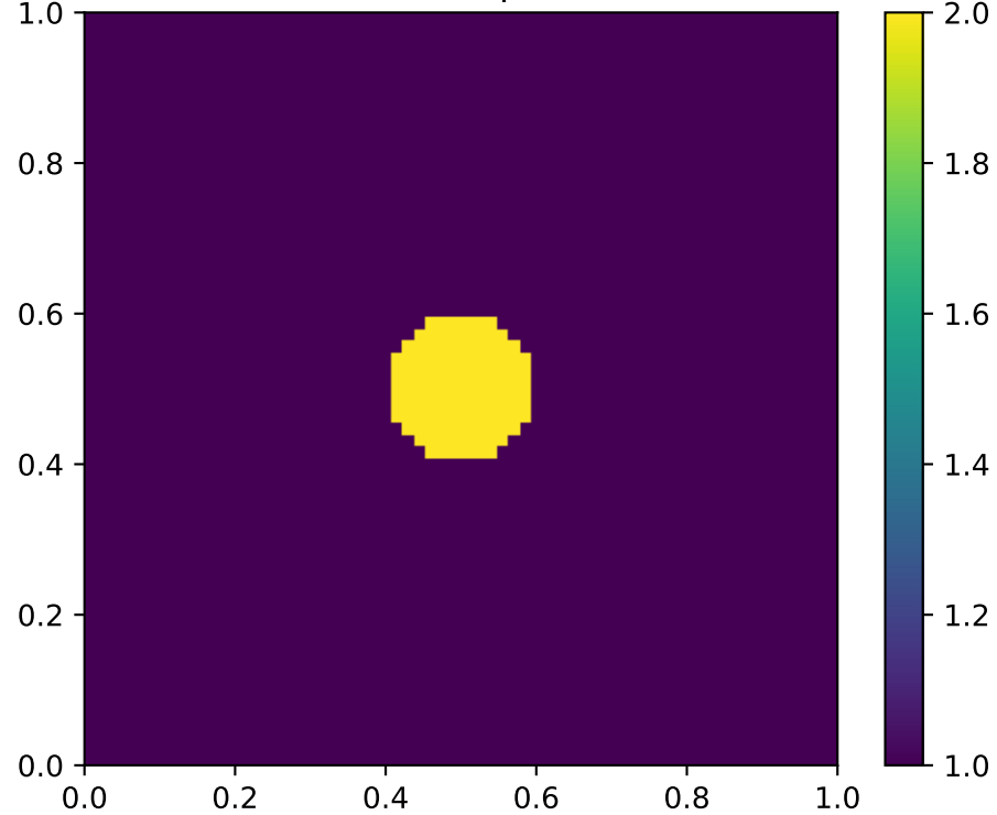
True \gamma
