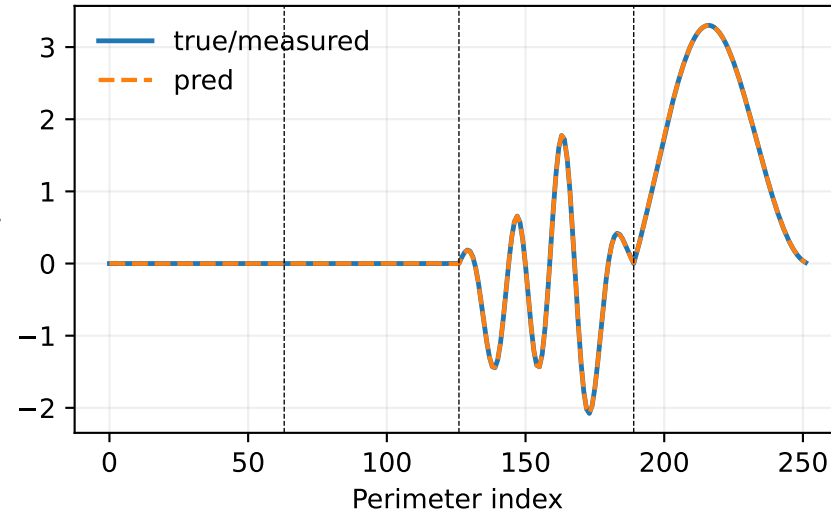
Dirichlet f_k ( k=49 )
