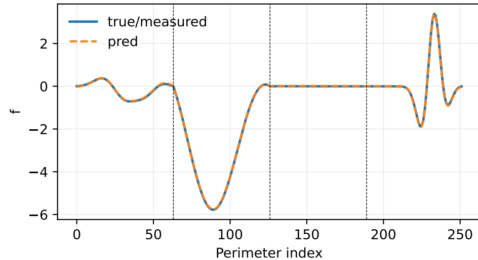
Dirichlet f_k (k=20)
