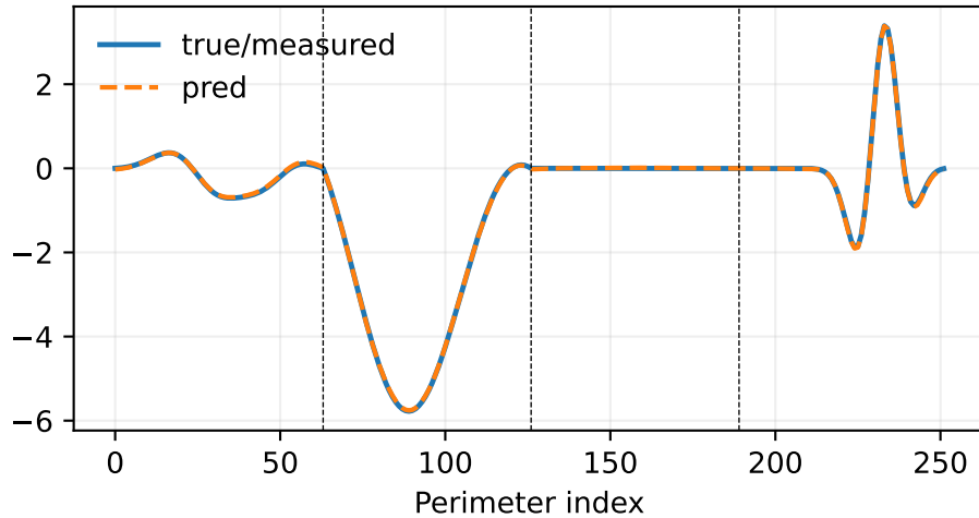
Dirichlet f_k (k=20)
