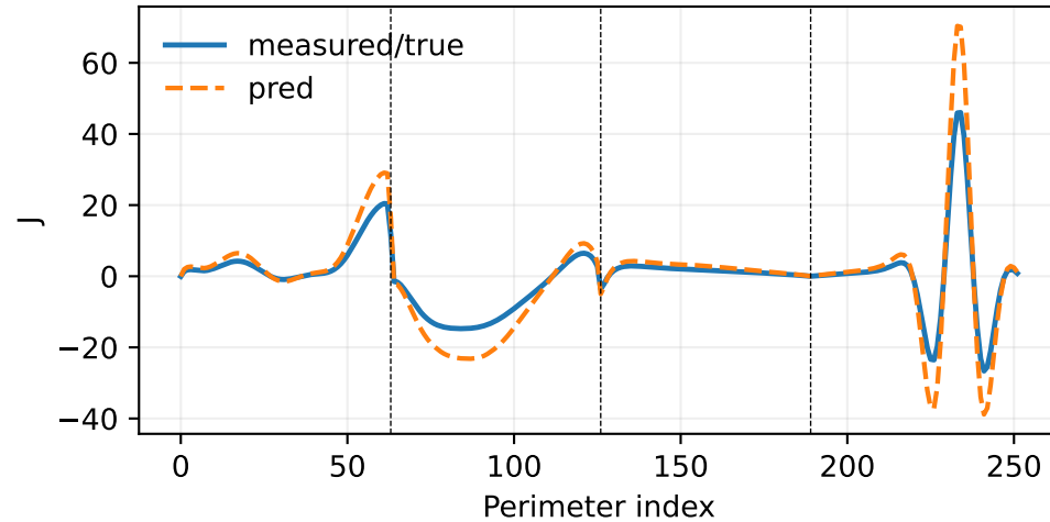
k=20 | RMS=5.10e+00 | max |\Delta J|=2.45e+01 Current J_k (k=20)
