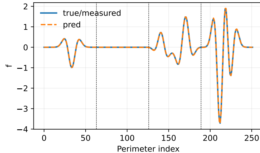
Dirichlet f_k ( k=10 )
