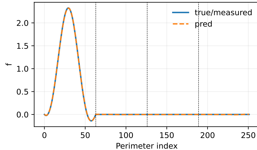
Dirichlet f_k (k=49)
