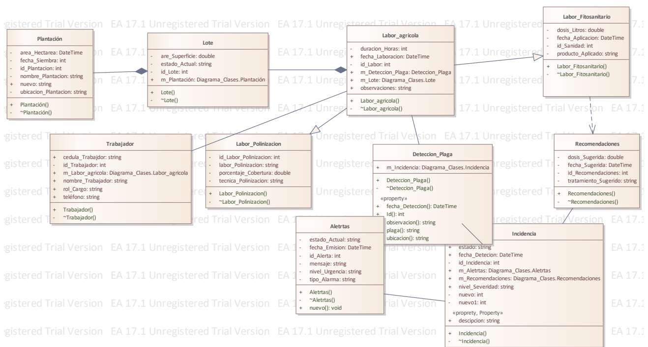
Figure 1: Diagrama_Clases
