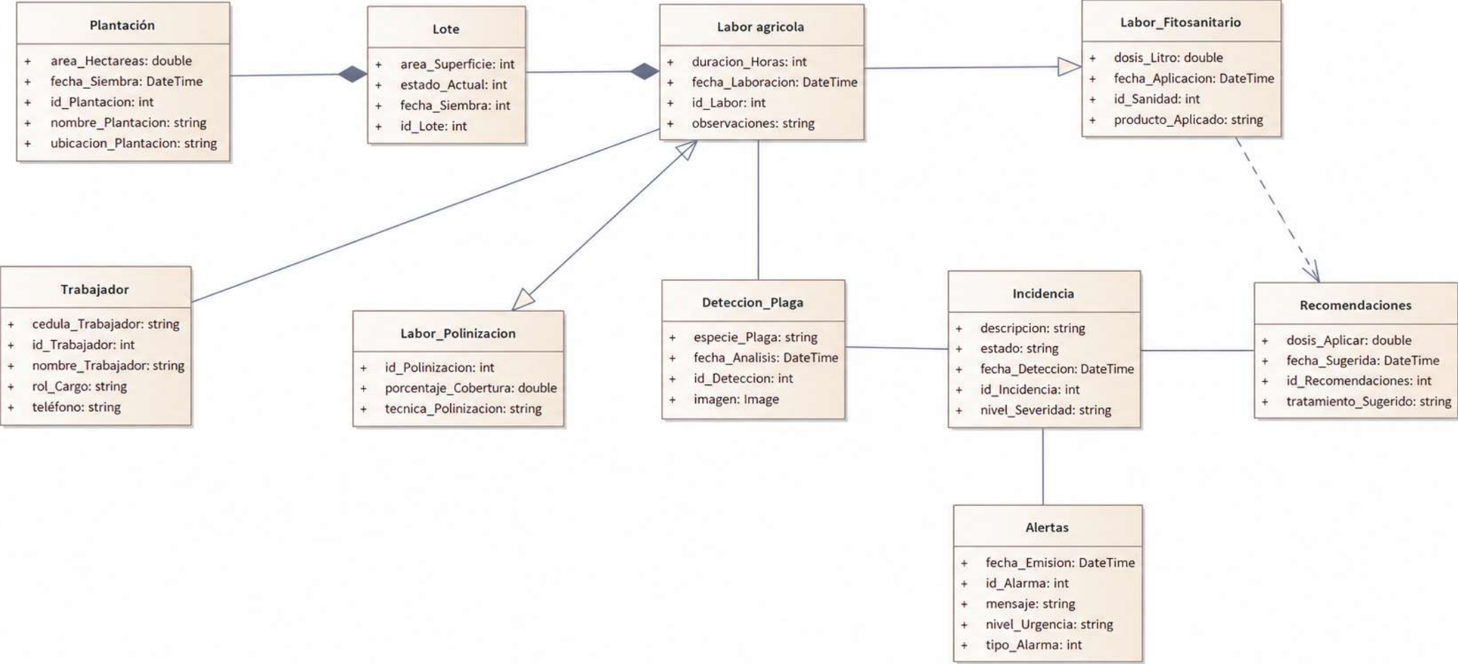
class Diagrama_Clases
