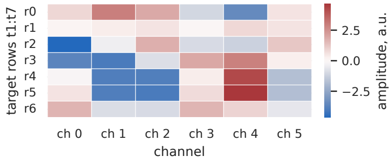
C. Target matrix slice Y
