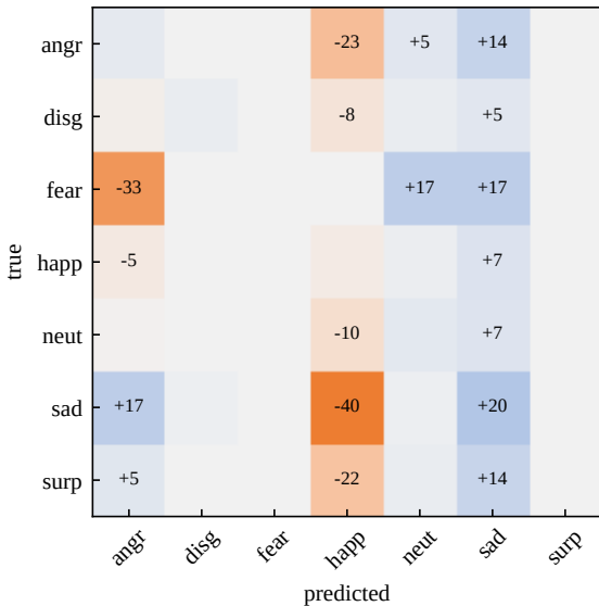
RoleNet – baseline (test, row %)
