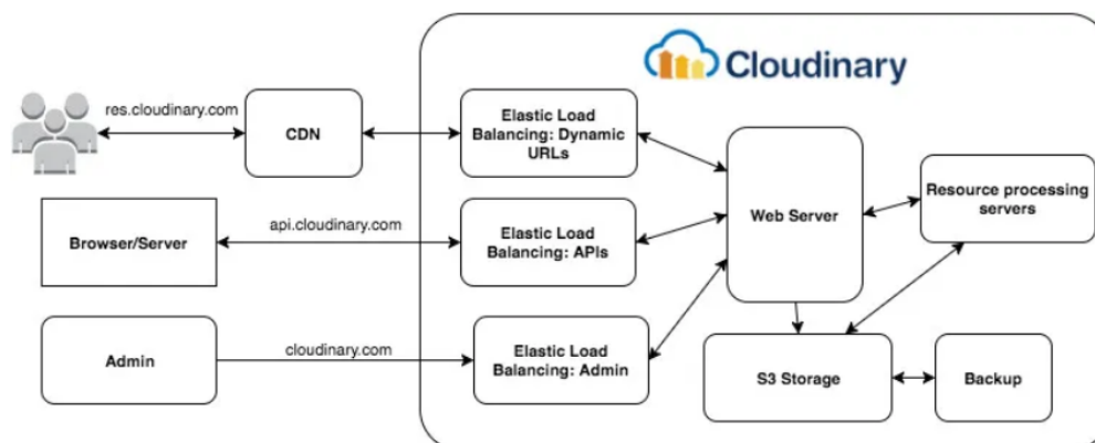
รูปที่ 2.10 ภาพรวม Service architecture ของ Cloudinary
