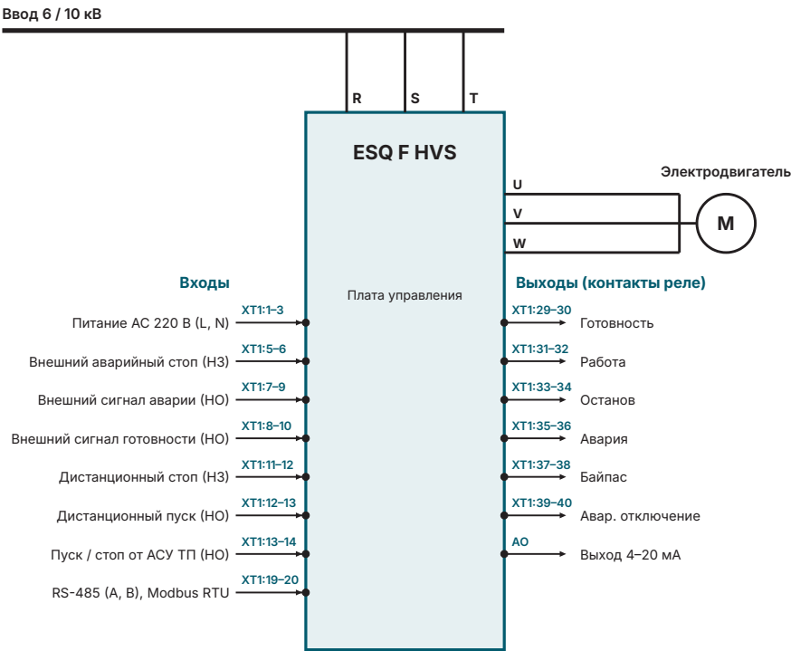
Рис. 9. Схема внешних подключений
