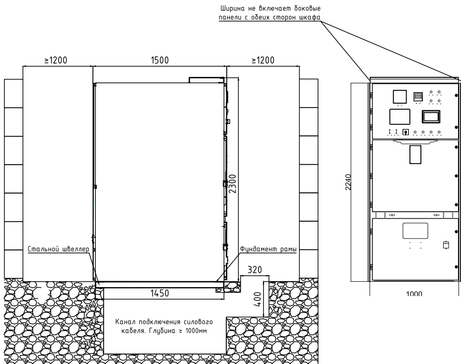
Рис. 10. Установочные размеры УПП (вид сбоку и вид спереди); ширина 1000 мм указана без боковых панелей
