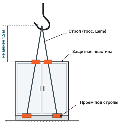
Рис. 4. Вид спереди при подъеме
