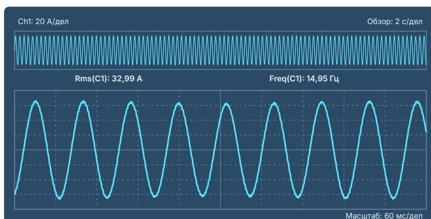
Рис. 3. Форма синусоидальной волны выходного тока.
