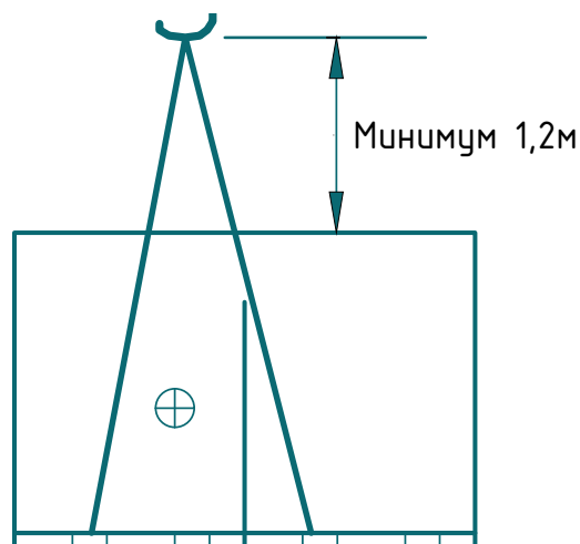
Рис. 4. Вид спереди при подъеме.
