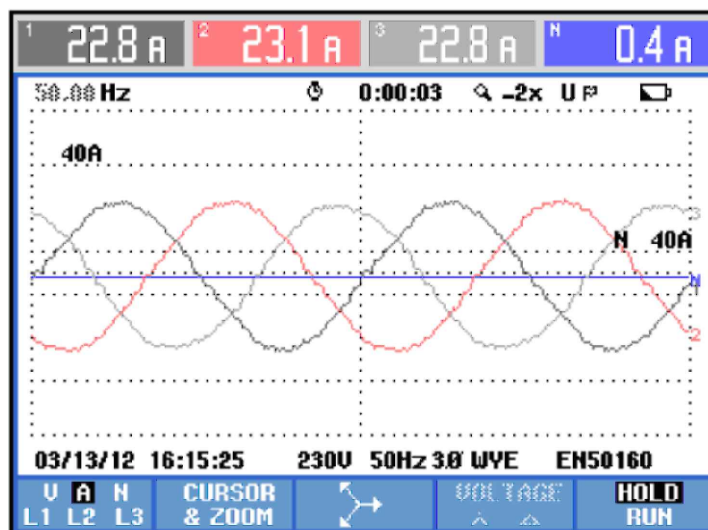
Рис. 1. Форма волны входного тока
