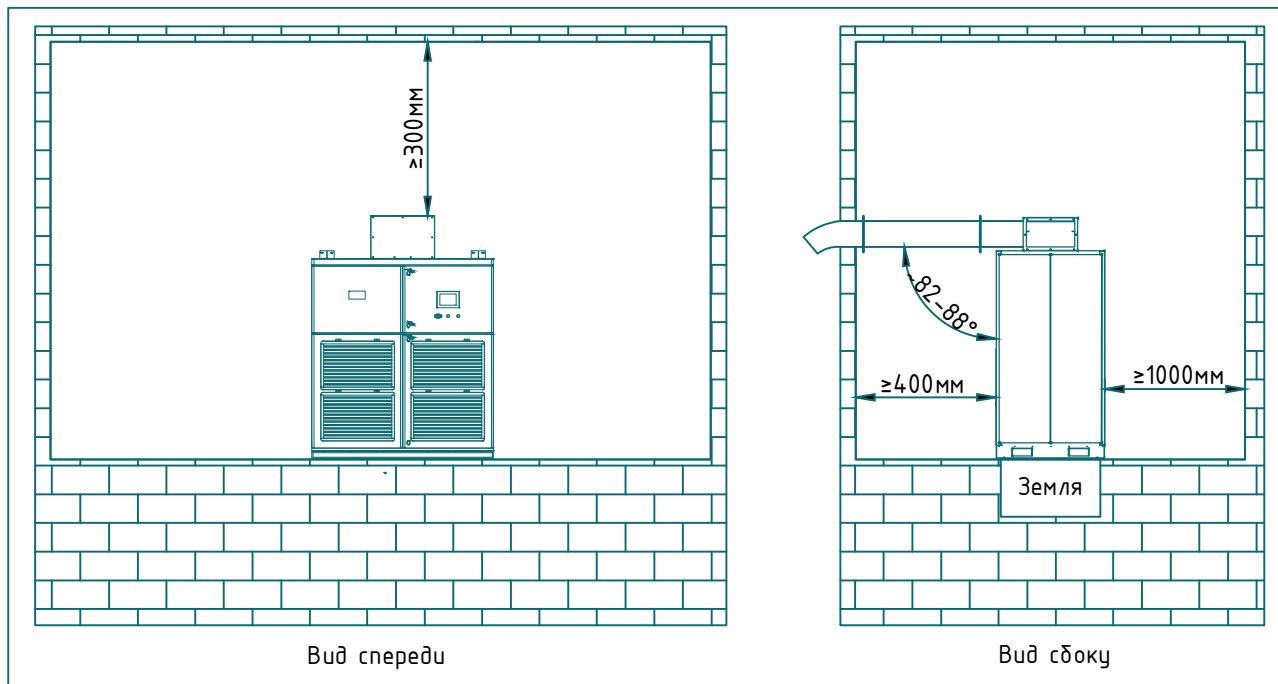
Рис. 6. Требования по установке.
