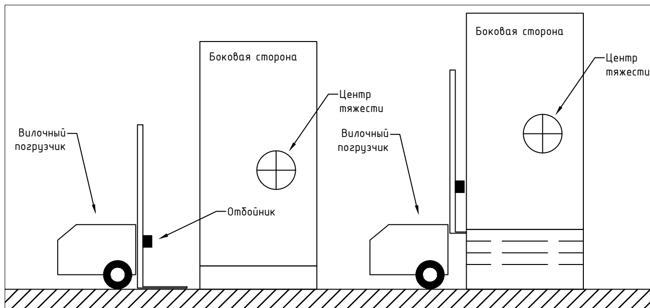
Рис. 5. Перемещение преобразователя при помощи автопогрузчика.
