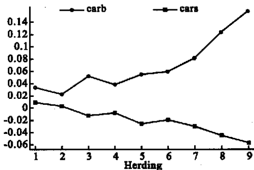
C. 羊群行为与同期收益(方法2)
