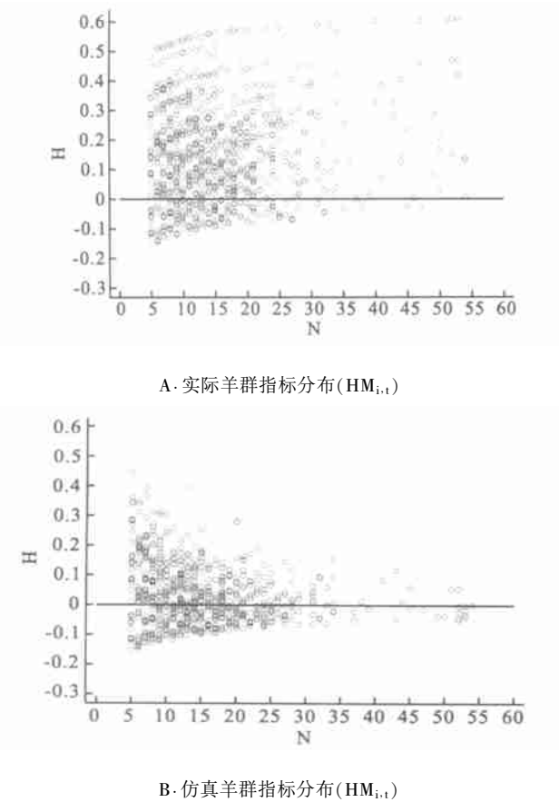
B. 仿真羊群指标分布( HM_{i,t}^* )
