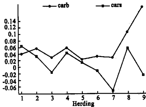
D. 羊群行为与后期收益
