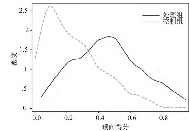
图 1 样本匹配前
