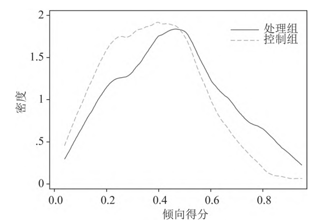
图 2 样本匹配后
