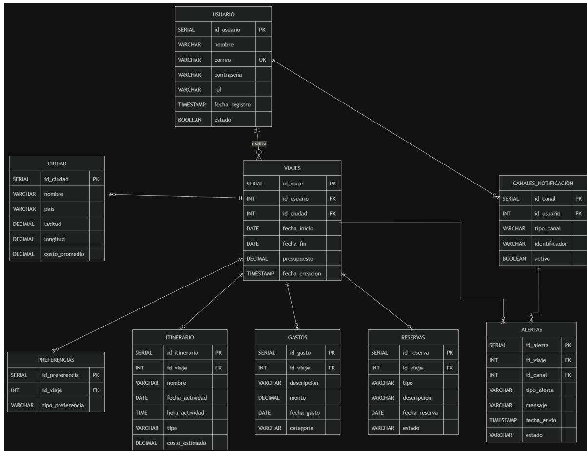
Figura 12. Evidencia de la implementación de la base de datos.
